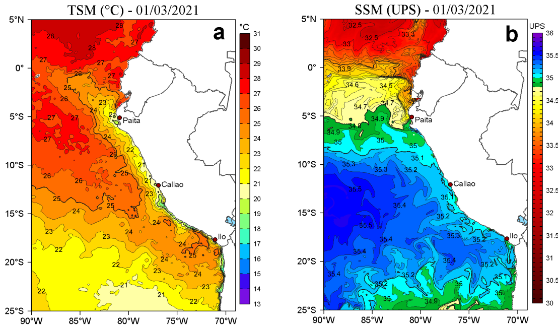
Figura 2. a) Temperatura superficial del mar (TSM, °C) y b) Salinidad superficial del mar (SSM) para el 01 de marzo de 2021. Datos: OSTIA-UKMO-L4-GLOB-v2.0 (UK Met Office, 2012; Donlon et al, 2012) disponible en https://podaac.jpl.nasa.gov/dataset/OSTIA-UKMO-L4-GLOB-v2.0 para (a) y Hybrid Coordinate Ocean Model v. GOFS 3.1 (HYCOM; Halliwell et al., 1998; 2000; Bleck, 2001) para (b).
