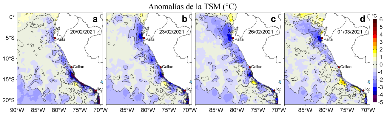
Figura 3. Anomalías de la temperatura superficial del mar (TSM, °C) para los días: a) 20, b) 23 y c) 26 de febrero y d) 01 de marzo de 2021. Las anomalías se calcularon respecto de la climatología para el periodo 2007-2016. Datos: OSTIA-UKMO-L4-GLOB-v2.0 (UK Met Office, 2012; Donlon et al, 2012).
