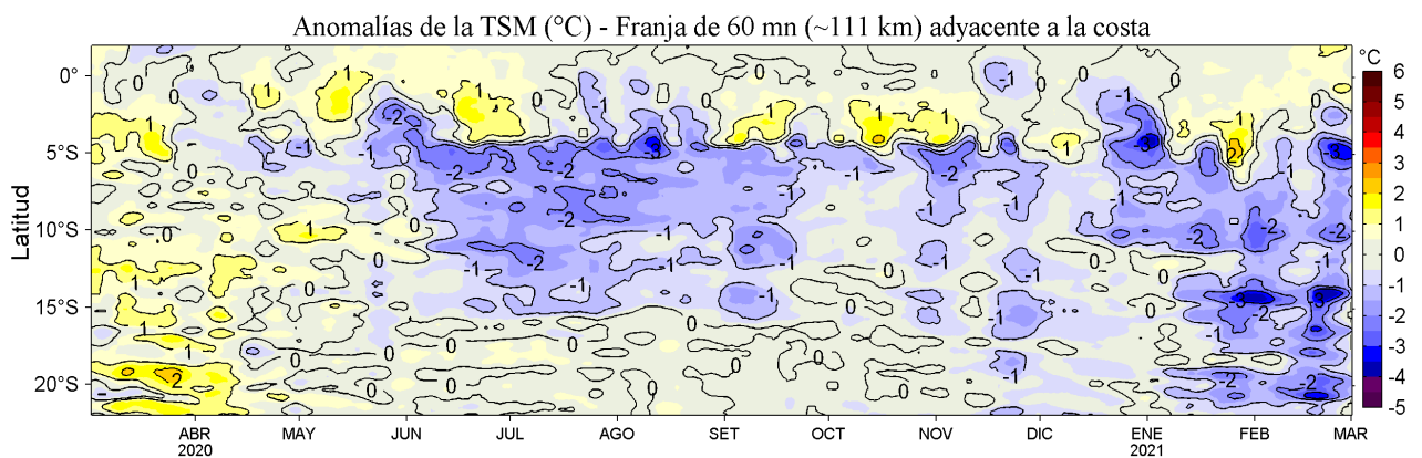
Figura 4. Variación promedio de las anomalías de la temperatura superficial del mar (TSM, °C) para una franja de 60 mn (~111 km) adyacente al litoral peruano para los últimos doce meses al 01 de marzo de 2021. Datos: OSTIA-UKMO-L4-GLOB-v2.0 (UK Met. Office, 2012; Donlon et al, 2012) disponible en https://podaac.jpl.nasa.gov/dataset/OSTIA-UKMO-L4-GLOB-v2.0 . Las anomalías se calcularon con respecto al periodo 2007-2016.
