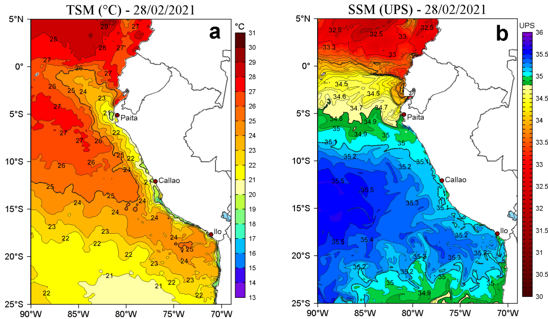
Figura 2. a) Temperatura superficial del mar (TSM, °C) y b) Salinidad superficial del mar (SSM) para el 28 de febrero de 2021. Datos: OSTIA-UKMO-L4-GLOB-v2.0 (UK Met Office, 2012; Donlon et al, 2012) disponible en https://podaac.jpl.nasa.gov/dataset/OSTIA-UKMO-L4-GLOB-v2.0 para (a) y Hybrid Coordinate Ocean Model v. GOF5 3.1 (HYCOM; Halliwell et al., 1998; 2000; Bleck, 2001) para (b).
