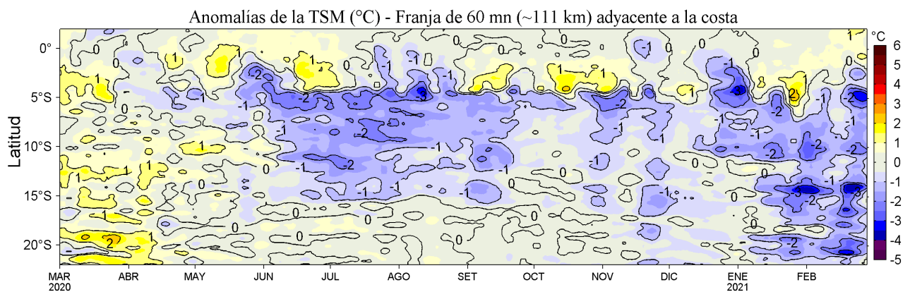
Figura 4. Variación promedio de las anomalías de la temperatura superficial del mar (TSM, °C) para una franja de 60 mn (~111 km) adyacente al litoral peruano para los últimos doce meses al 28 de febrero de 2021. Datos: OSTIA-UKMO-L4-GLOB-v2.0 (UK Met. Office, 2012; Donlon et al, 2012) disponible en https://podaac.jpl.nasa.gov/dataset/OSTIA-UKMO-L4-GLOB-v2.0 . Las anomalías se calcularon con respecto al periodo 2007-2016.
