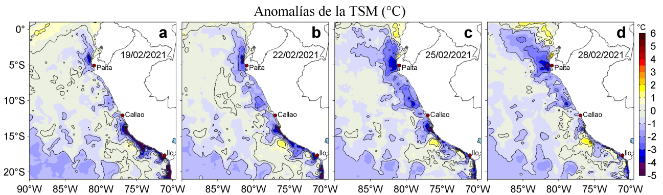
Figura 3. Anomalías de la temperatura superficial del mar (TSM, °C) para los días: a) 19, b) 22, c) 25 y d) 28 de febrero de 2021. Las anomalías se calcularon respecto de la climatología para el periodo 2007-2016. Datos: OSTIA-UKMO-L4-GLOB-v2.0 (UK Met Office, 2012; Donlon et al, 2012).
