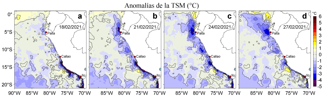
Figura 3. Anomalías de la temperatura superficial del mar (TSM, °C) para los días: a) 18, b) 21, c) 24 y d) 27 de febrero de 2021. Las anomalías se calcularon respecto de la climatología para el periodo 2007-2016. Datos: OSTIA-UKMO-L4-GLOB-v2.0 (UK Met Office, 2012; Donlon et al, 2012).
