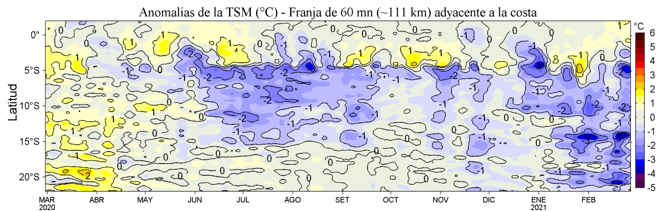
Figura 4. Variación promedio de las anomalías de la temperatura superficial del mar (TSM, °C) para una franja de 60 mn (~111 km) adyacente al litoral peruano para los últimos doce meses al 27 de febrero de 2021. Datos: OSTIA-UKMO-L4-GLOB-v2.0 (UK Met. Office, 2012; Donlon et al, 2012) disponible en https://podaac.jpl.nasa.gov/dataset/OSTIA-UKMO-L4-GLOB-v2.0 . Las anomalías se calcularon con respecto al periodo 2007-2016.
