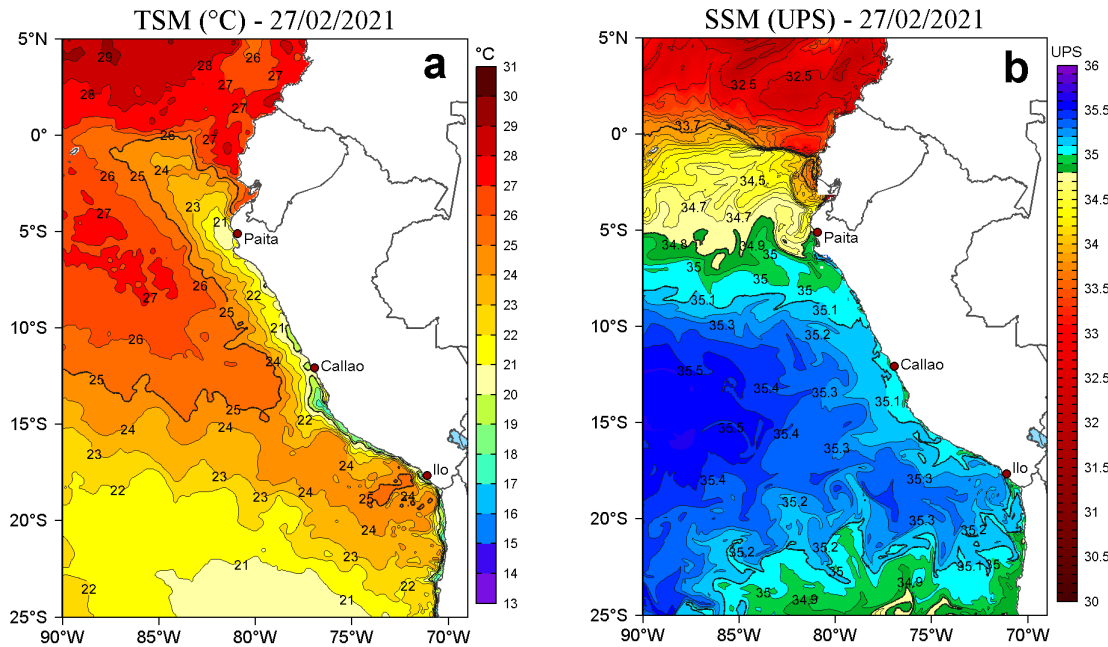
Figura 2. a) Temperatura superficial del mar (TSM, °C) y b) Salinidad superficial del mar (SSM) para el 27 de febrero de 2021. Datos: OSTIA-UKMO-L4-GLOB-v2.0 (UK Met Office, 2012; Donlon et al, 2012) disponible en https://podaac.jpl.nasa.gov/dataset/OSTIA-UKMO-L4-GLOB-v2.0 para (a) y Hybrid Coordinate Ocean Model v. GOF5 3.1 (HYCOM; Halliwell et al., 1998; 2000; Bleck, 2001) para (b).
