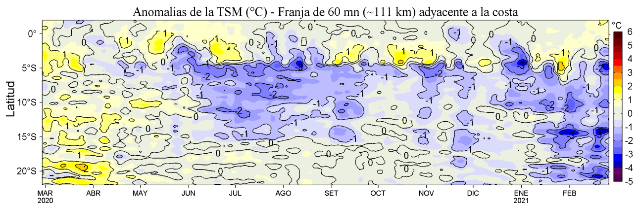
Figura 4. Variación promedio de las anomalías de la temperatura superficial del mar (TSM, °C) para una franja de 60 mn (~111 km) adyacente al litoral peruano para los últimos doce meses al 26 de febrero de 2021. Datos: OSTIA-UKMO-L4-GLOB-v2.0 (UK Met. Office, 2012; Donlon et al, 2012) disponible en https://podaac.jpl.nasa.gov/dataset/OSTIA-UKMO-L4-GLOB-v2.0 . Las anomalías se calcularon con respecto al periodo 2007-2016.
