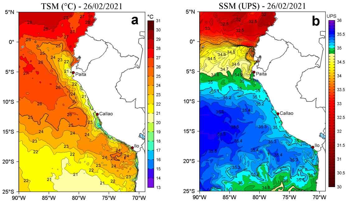
Figura 2. a) Temperatura superficial del mar (TSM, °C) y b) Salinidad superficial del mar (SSM) para el 26 de febrero de 2021. Datos: OSTIA-UKMO-L4-GLOB-v2.0 (UK Met Office, 2012; Donlon et al, 2012) disponible en https://podaac.jpl.nasa.gov/dataset/OSTIA-UKMO-L4-GLOB-v2.0 para (a) y Hybrid Coordinate Ocean Model v. GOF5 3.1 (HYCOM; Halliwell et al., 1998; 2000; Bleck, 2001) para (b).
