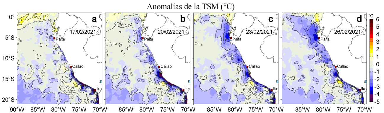
Figura 3. Anomalías de la temperatura superficial del mar (TSM, °C) para los días: a) 17, b) 20, c) 23 y d) 26 de febrero de 2021. Las anomalías se calcularon respecto de la climatología para el periodo 2007-2016. Datos: OSTIA-UKMO-L4-GLOB-v2.0 (UK Met Office, 2012; Donlon et al, 2012).
