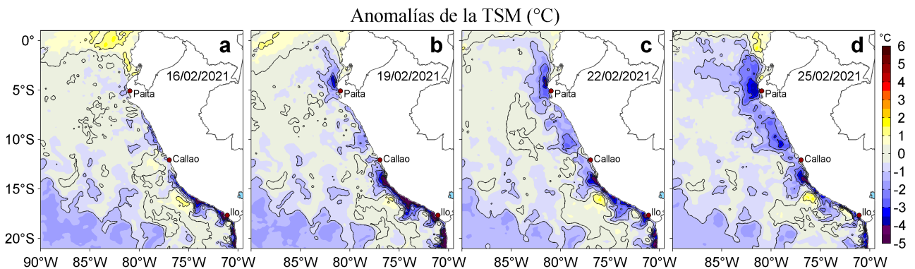
Figura 3. Anomalías de la temperatura superficial del mar (TSM, °C) para los días: a) 16, b) 19, c) 22 y d) 25 de febrero de 2021. Las anomalías se calcularon respecto de la climatología para el periodo 2007-2016. Datos: OSTIA-UKMO-L4-GLOB-v2.0 (UK Met Office, 2012; Donlon et al, 2012).
