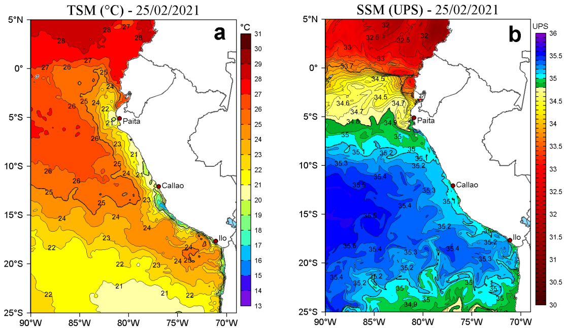
Figura 2. a) Temperatura superficial del mar (TSM, °C) y b) Salinidad superficial del mar (SSM) para el 25 de febrero de 2021. Datos: OSTIA-UKMO-L4-GLOB-v2.0 (UK Met Office, 2012; Donlon et al, 2012) disponible en https://podaac.jpl.nasa.gov/dataset/OSTIA-UKMO-L4-GLOB-v2.0 para (a) y Hybrid Coordinate Ocean Model v. GOF5 3.1 (HYCOM; Halliwell et al., 1998; 2000; Bleck, 2001) para (b).
