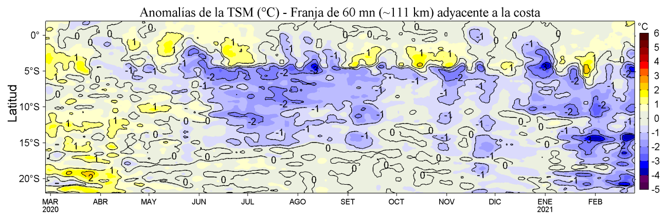
Figura 4. Variación promedio de las anomalías de la temperatura superficial del mar (TSM, °C) para una franja de 60 mn (~111 km) adyacente al litoral peruano para los últimos doce meses al 25 de febrero de 2021. Datos: OSTIA-UKMO-L4-GLOB-v2.0 (UK Met. Office, 2012; Donlon et al, 2012) disponible en https://podaac.jpl.nasa.gov/dataset/OSTIA-UKMO-L4-GLOB-v2.0 . Las anomalías se calcularon con respecto al periodo 2007-2016.
