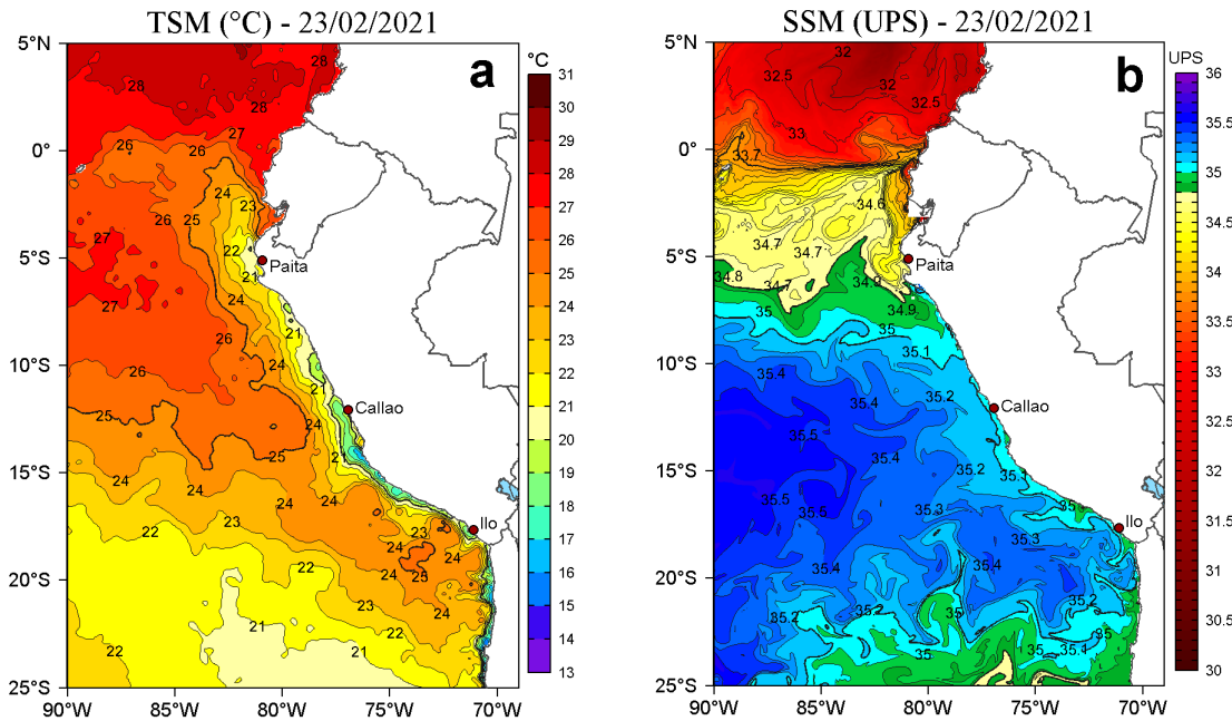
Figura 2. a) Temperatura superficial del mar (TSM, °C) y b) Salinidad superficial del mar (SSM) para el 23 de febrero de 2021. Datos: OSTIA-UKMO-L4-GLOB-v2.0 (UK Met Office, 2012; Donlon et al, 2012) disponible en https://podaac.jpl.nasa.gov/dataset/OSTIA-UKMO-L4-GLOB-v2.0 para (a) y Hybrid Coordinate Ocean Model v. GOFS 3.1 (HYCOM; Halliwell et al., 1998; 2000; Bleck, 2001) para (b).
