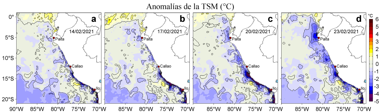
Figura 3. Anomalías de la temperatura superficial del mar (TSM, °C) para los días: a) 14, b) 17, c) 20 y d) 23 de febrero de 2021. Las anomalías se calcularon respecto de la climatología para el periodo 2007-2016. Datos: OSTIA-UKMO-L4-GLOB-v2.0 (UK Met Office, 2012; Donlon et al, 2012).
