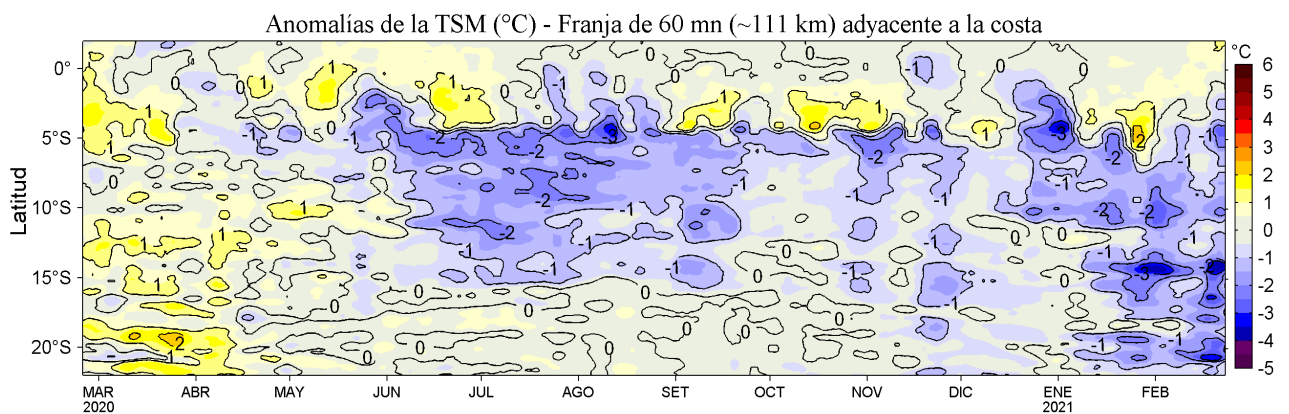
Figura 4. Variación promedio de las anomalías de la temperatura superficial del mar (TSM, °C) para una franja de 60 mn (~111 km) adyacente al litoral peruano para los últimos doce meses al 23 de febrero de 2021. Datos: OSTIA-UKMO-L4-GLOB-v2.0 (UK Met. Office, 2012; Donlon et al, 2012) disponible en https://podaac.jpl.nasa.gov/dataset/OSTIA-UKMO-L4-GLOB-v2.0 . Las anomalías se calcularon con respecto al periodo 2007-2016.
