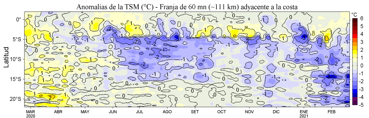
Figura 4. Variación promedio de las anomalías de la temperatura superficial del mar (TSM, °C) para una franja de 60 mn (~111 km) adyacente al litoral peruano para los últimos doce meses al 21 de febrero de 2021. Datos: OSTIA-UKMO-L4-GLOB-v2.0 (UK Met. Office, 2012; Donlon et al, 2012) disponible en https://podaac.jpl.nasa.gov/dataset/OSTIA-UKMO-L4-GLOB-v2.0 . Las anomalías se calcularon con respecto al periodo 2007-2016.
