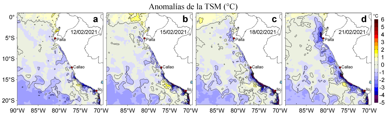
Figura 3. Anomalías de la temperatura superficial del mar (TSM, °C) para los días: a) 12, b) 15, c) 18 y d) 21 de febrero de 2021. Las anomalías se calcularon respecto de la climatología para el periodo 2007-2016. Datos: OSTIA-UKMO-L4-GLOB-v2.0 (UK Met Office, 2012; Donlon et al, 2012).
