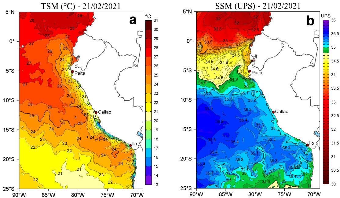
Figura 2. a) Temperatura superficial del mar (TSM, °C) y b) Salinidad superficial del mar (SSM) para el 21 de febrero de 2021. Datos: OSTIA-UKMO-L4-GLOB-v2.0 (UK Met Office, 2012; Donlon et al, 2012) disponible en https://podaac.jpl.nasa.gov/dataset/OSTIA-UKMO-L4-GLOB-v2.0 para (a) y Hybrid Coordinate Ocean Model v. GOFS 3.1 (HYCOM; Halliwell et al., 1998; 2000; Bleck, 2001) para (b).
