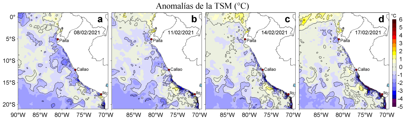
Figura 3. Anomalías de la temperatura superficial del mar (TSM, °C) para los días: a) 08, b) 11, c) 14 y d) 17 de febrero de 2021. Las anomalías se calcularon respecto de la climatología para el periodo 2007-2016. Datos: OSTIA-UKMO-L4-GLOB-v2.0 (UK Met Office, 2012; Donlon et al, 2012).
