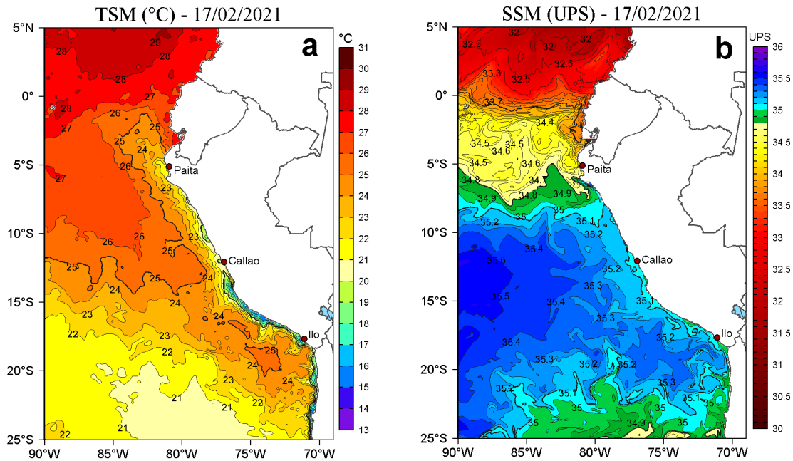
Figura 2. a) Temperatura superficial del mar (TSM, °C) y b) Salinidad superficial del mar (SSM) para el 17 de febrero de 2021. Datos: OSTIA-UKMO-L4-GLOB-v2.0 (UK Met Office, 2012; Donlon et al, 2012) disponible en https://podaac.jpl.nasa.gov/dataset/OSTIA-UKMO-L4-GLOB-v2.0 para (a) y Hybrid Coordinate Ocean Model v. GOFS 3.1 (HYCOM; Halliwell et al., 1998; 2000; Bleck, 2001) para (b).
