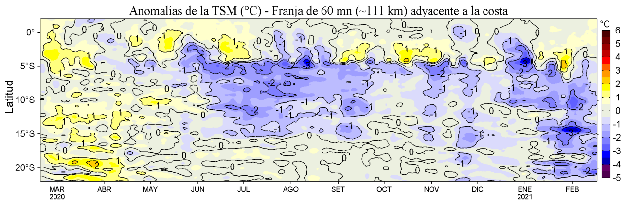
Figura 4. Variación promedio de las anomalías de la temperatura superficial del mar (TSM, °C) para una franja de 60 mn (~111 km) adyacente al litoral peruano para los últimos doce meses al 17 de febrero de 2021. Datos: OSTIA-UKMO-L4-GLOB-v2.0 (UK Met. Office, 2012; Donlon et al, 2012) disponible en https://podaac.jpl.nasa.gov/dataset/OSTIA-UKMO-L4-GLOB-v2.0 . Las anomalías se calcularon con respecto al periodo 2007-2016.
