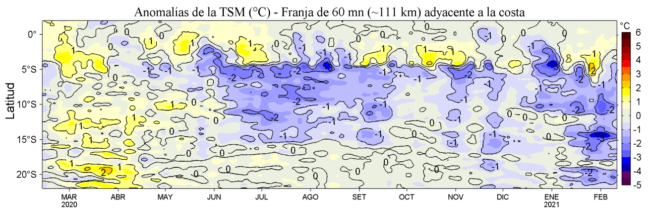
Figura 4. Variación promedio de las anomalías de la temperatura superficial del mar (TSM, °C) para una franja de 60 mn (~111 km) adyacente al litoral peruano para los últimos doce meses al 11 de febrero de 2021. Datos: OSTIA-UKMO-L4-GLOB-v2.0 (UK Met. Office, 2012; Donlon et al, 2012) disponible en https://podaac.jpl.nasa.gov/dataset/OSTIA-UKMO-L4-GLOB-v2.0 . Las anomalías se calcularon con respecto al periodo 2007-2016.
