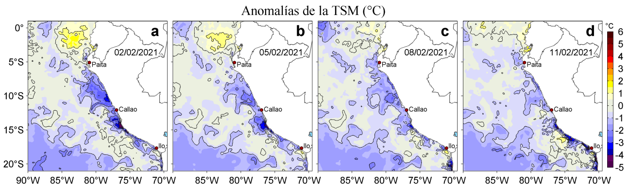
Figura 3. Anomalías de la temperatura superficial del mar (TSM, °C) para los días: a) 02, b) 05, c) 08 y d) 11 de febrero de 2021. Las anomalías se calcularon respecto de la climatología para el periodo 2007-2016. Datos: OSTIA-UKMO-L4-GLOB-v2.0 (UK Met Office, 2012; Donlon et al, 2012).
