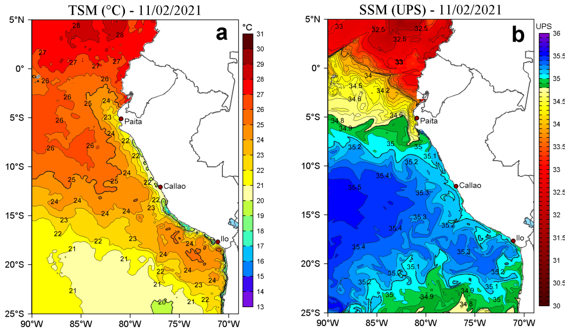
Figura 2. a) Temperatura superficial del mar (TSM, °C) y b) Salinidad superficial del mar (SSM) para el 11 de febrero de 2021. Datos: OSTIA-UKMO-L4-GLOB-v2.0 (UK Met Office, 2012; Donlon et al, 2012) disponible en https://podaac.jpl.nasa.gov/dataset/OSTIA-UKMO-L4-GLOB-v2.0 para (a) y Hybrid Coordinate Ocean Model v. GOF5 3.1 (HYCOM; Halliwell et al., 1998; 2000; Bleck, 2001) para (b).
