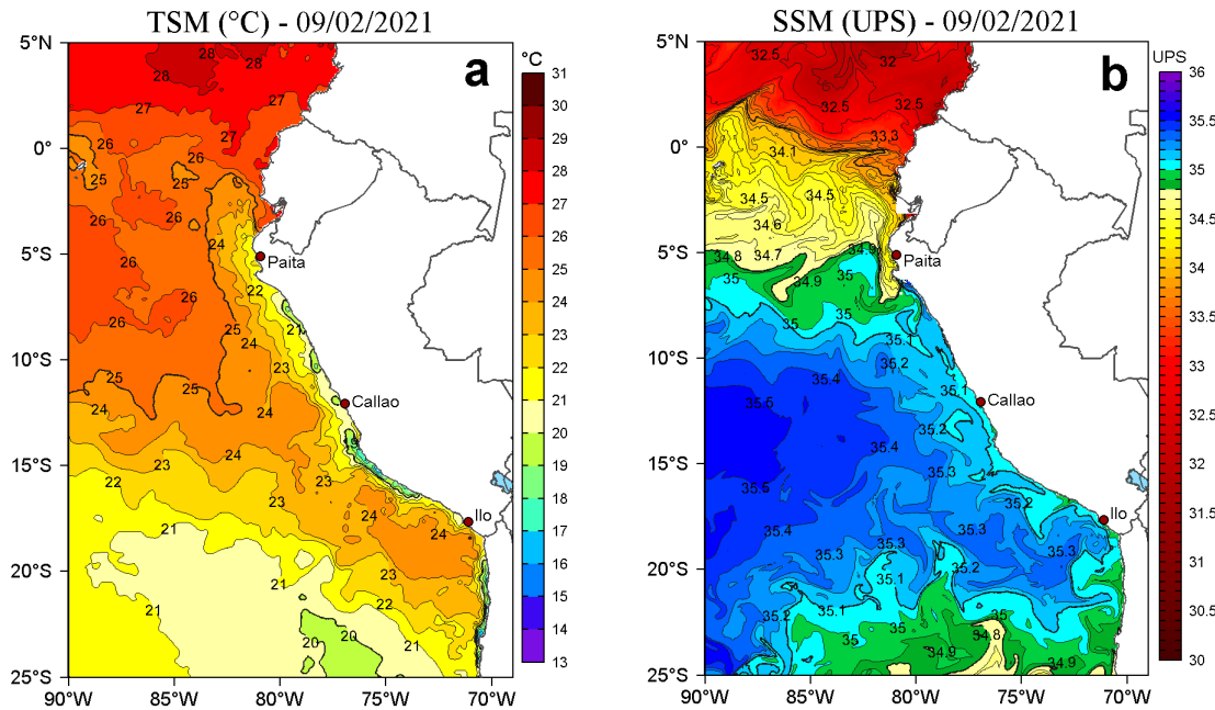
Figura 2. a) Temperatura superficial del mar (TSM, °C) y b) Salinidad superficial del mar (SSM) para el 09 de febrero de 2021. Datos: OSTIA-UKMO-L4-GLOB-v2.0 (UK Met Office, 2012; Donlon et al, 2012) disponible en https://podaac.jpl.nasa.gov/dataset/OSTIA-UKMO-L4-GLOB-v2.0 para (a) y Hybrid Coordinate Ocean Model v. GOFS 3.1 (HYCOM; Halliwell et al., 1998; 2000; Bleck, 2001) para (b).
