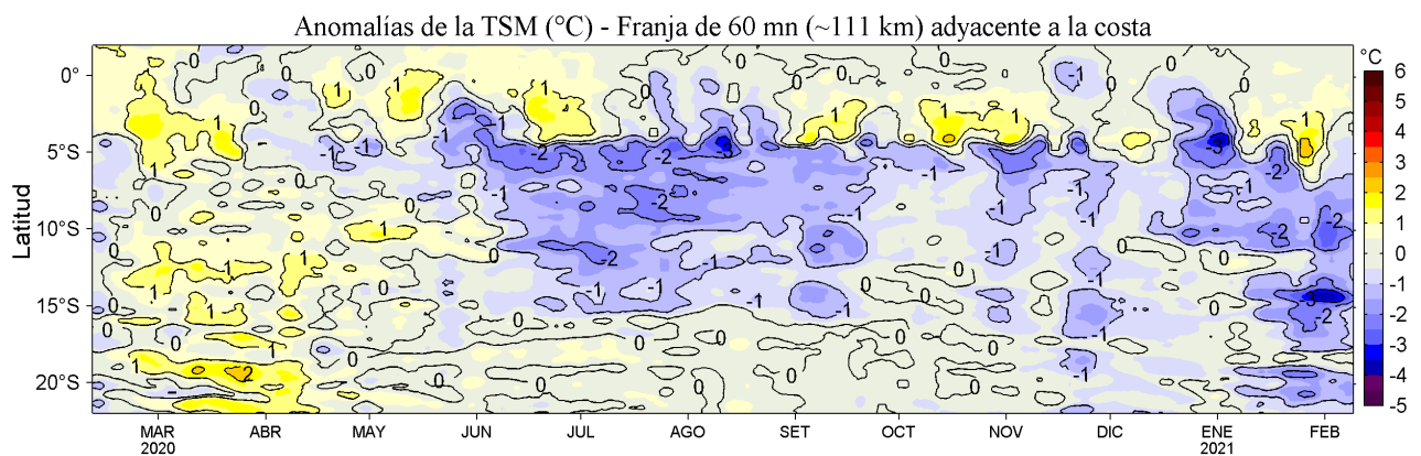
Figura 4. Variación promedio de las anomalías de la temperatura superficial del mar (TSM, °C) para una franja de 60 mn (~111 km) adyacente al litoral peruano para los últimos doce meses al 09 de febrero de 2021. Datos: OSTIA-UKMO-L4-GLOB-v2.0 (UK Met. Office, 2012; Donlon et al, 2012) disponible en https://podaac.jpl.nasa.gov/dataset/OSTIA-UKMO-L4-GLOB-v2.0 . Las anomalías se calcularon con respecto al periodo 2007-2016.
