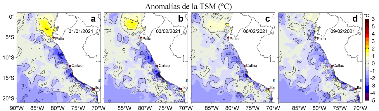
Figura 3. Anomalías de la temperatura superficial del mar (TSM, °C) para los días: a) 31 de enero, b) 03, c) 06 y d) 09 de febrero de 2021. Las anomalías se calcularon respecto de la climatología para el periodo 2007-2016. Datos: OSTIA-UKMO-L4-GLOB-v2.0 (UK Met Office, 2012; Donlon et al, 2012).
