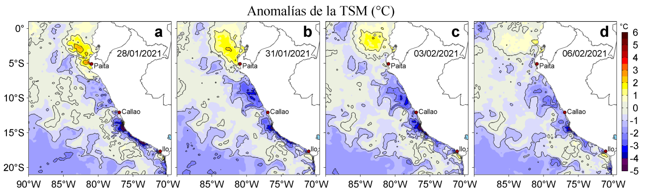
Figura 3. Anomalías de la temperatura superficial del mar (TSM, °C) para los días: a) 28 y b) 31 de enero, c) 03 y d) 06 de febrero de 2021. Las anomalías se calcularon respecto de la climatología para el periodo 2007-2016. Datos: OSTIA-UKMO-L4-GLOB-v2.0 (UK Met Office, 2012; Donlon et al, 2012).
