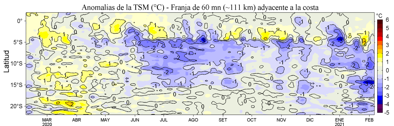
Figura 4. Variación promedio de las anomalías de la temperatura superficial del mar (TSM, °C) para una franja de 60 mn (~111 km) adyacente al litoral peruano para los últimos doce meses al 06 de febrero de 2021. Datos: OSTIA-UKMO-L4-GLOB-v2.0 (UK Met. Office, 2012; Donlon et al, 2012) disponible en https://podaac.jpl.nasa.gov/dataset/OSTIA-UKMO-L4-GLOB-v2.0 . Las anomalías se calcularon con respecto al periodo 2007-2016.
