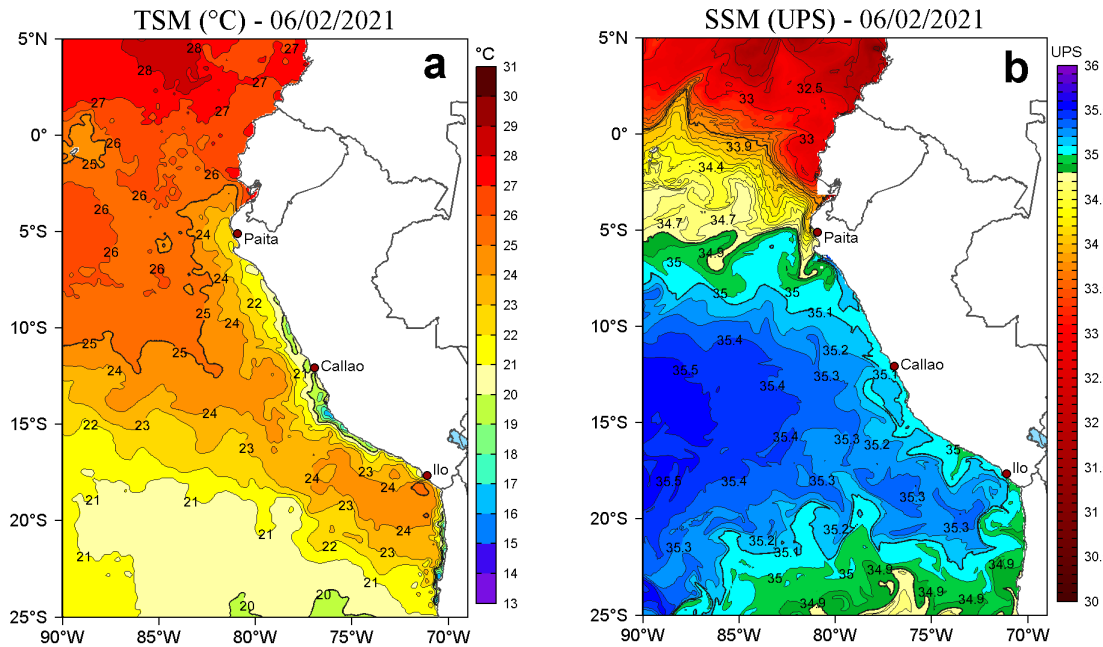
Figura 2. a) Temperatura superficial del mar (TSM, °C) y b) Salinidad superficial del mar (SSM) para el 06 de febrero de 2021. Datos: OSTIA-UKMO-L4-GLOB-v2.0 (UK Met Office, 2012; Donlon et al, 2012) disponible en https://podaac.jpl.nasa.gov/dataset/OSTIA-UKMO-L4-GLOB-v2.0 para (a) y Hybrid Coordinate Ocean Model v. GOF5 3.1 (HYCOM; Halliwell et al., 1998; 2000; Bleck, 2001) para (b).
