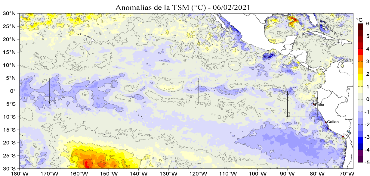
Figura 1. Anomalías de la temperatura superficial del mar (TSM, °C) en el océano Pacífico tropical. Las regiones Niño 3.4 (5°N - 5°S, 170°W - 120°W) y Niña 1+2 (0 - 10°S, 90°W - 80°W) en los sectores central y oriental del océano, respectivamente, están delimitadas con una línea de color negro. Las anomalías se estimaron de acuerdo a la climatología para el periodo 2007-2016. Los datos provienen de OSTIA-UKMO-L4-GLOB-v2.0 (UK Met Office, 2012; Donlon et al, 2012) y están disponibles en https://podaac.jpl.nasa.gov/dataset/OSTIA-UKMO-L4-GLOB-v2.0 .
