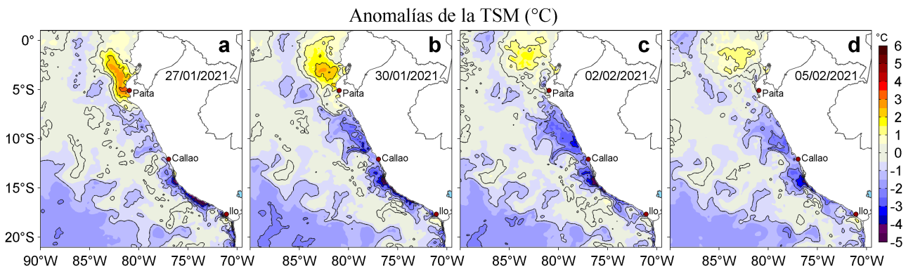
Figura 3. Anomalías de la temperatura superficial del mar (TSM, °C) para los días: a) 27 y b) 30 de enero, c) 02 y d) 05 de febrero de 2021. Las anomalías se calcularon respecto de la climatología para el periodo 2007-2016. Datos: OSTIA-UKMO-L4-GLOB-v2.0 (UK Met Office, 2012; Donlon et al, 2012).
