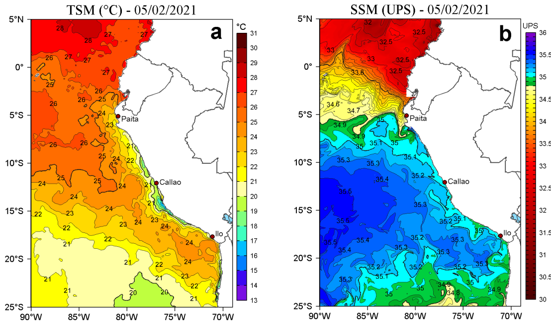
Figura 2. a) Temperatura superficial del mar (TSM, °C) y b) Salinidad superficial del mar (SSM) para el 05 de febrero de 2021. Datos: OSTIA-UKMO-L4-GLOB-v2.0 (UK Met Office, 2012; Donlon et al, 2012) disponible en https://podaac.jpl.nasa.gov/dataset/OSTIA-UKMO-L4-GLOB-v2.0 para (a) y Hybrid Coordinate Ocean Model v. GOFS 3.1 (HYCOM; Halliwell et al., 1998; 2000; Bleck, 2001) para (b).
