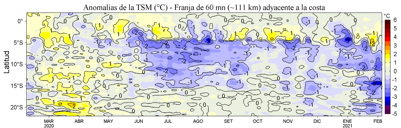
Figura 4. Variación promedio de las anomalías de la temperatura superficial del mar (TSM, °C) para una franja de 60 mn (~111 km) adyacente al litoral peruano para los últimos doce meses al 05 de febrero de 2021. Datos: OSTIA-UKMO-L4-GLOB-v2.0 (UK Met. Office, 2012; Donlon et al, 2012) disponible en https://podaac.jpl.nasa.gov/dataset/OSTIA-UKMO-L4-GLOB-v2.0 . Las anomalías se calcularon con respecto al periodo 2007-2016.
