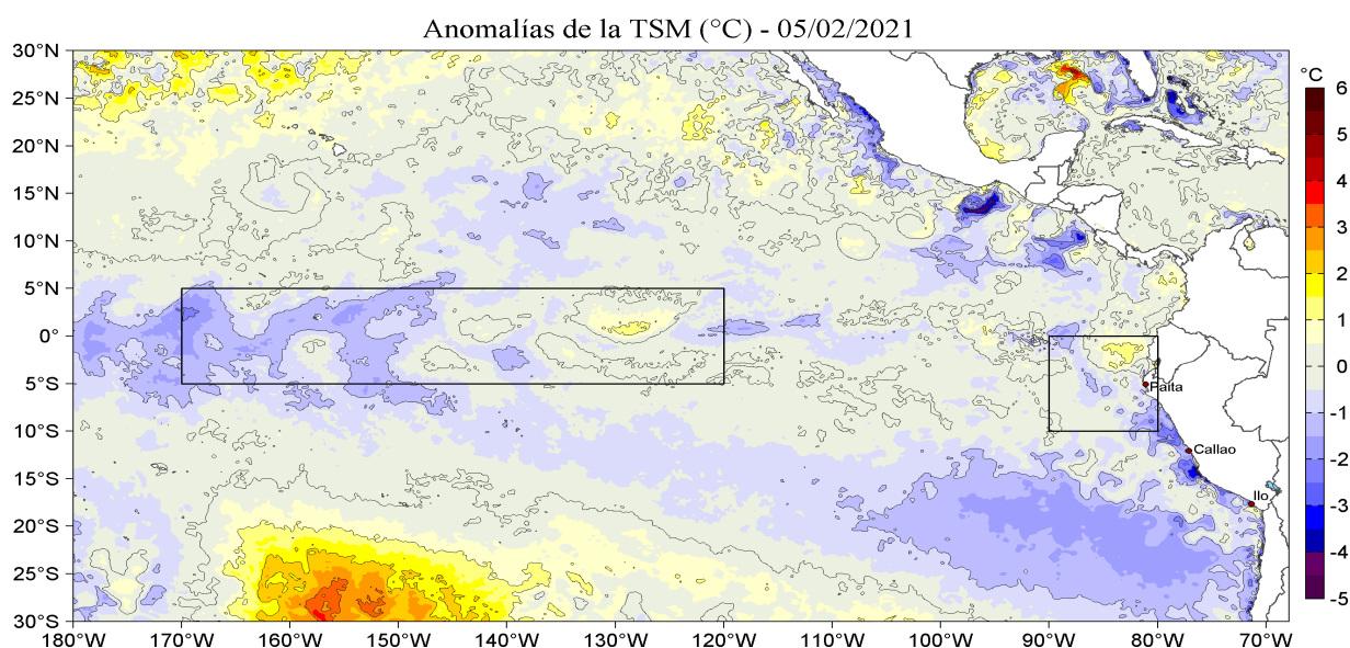
Figura 1. Anomalías de la temperatura superficial del mar (TSM, °C) en el océano Pacífico tropical. Las regiones Niño 3.4 (5 °N - 5 °S, 170 °W - 120 °W) y Niña 1+2 (0 - 10 °S, 90 °W - 80 °W) en los sectores central y oriental del océano, respectivamente, están delimitadas con una línea de color negro. Las anomalías se estimaron de acuerdo a la climatología para el periodo 2007-2016. Los datos provienen de OSTIA-UKMO-L4-GLOB-v2.0 (UK Met Office, 2012; Donlon et al, 2012) y están disponibles en https://podaac.jpl.nasa.gov/dataset/OSTIA-UKMO-L4-GLOB-v2.0 .
