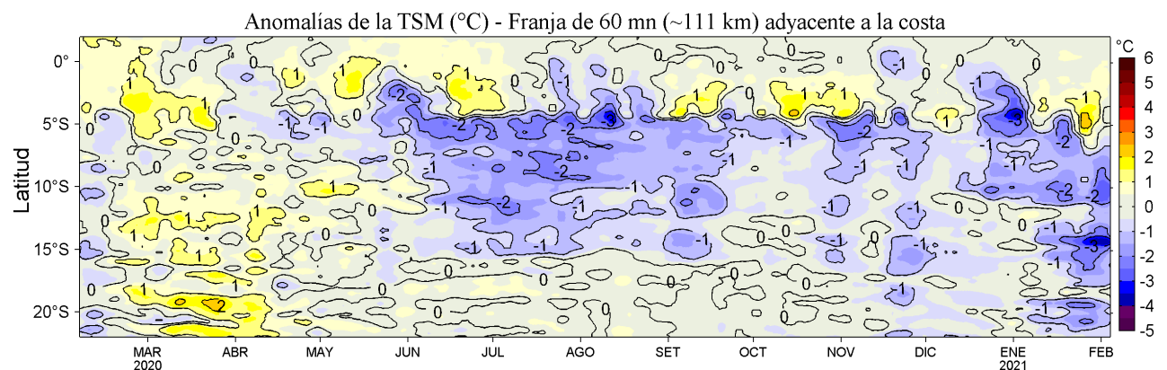
Figura 4. Variación promedio de las anomalías de la temperatura superficial del mar (TSM, °C) para una franja de 60 mn (~111 km) adyacente al litoral peruano para los últimos doce meses al 04 de febrero de 2021. Datos: OSTIA-UKMO-L4-GLOB-v2.0 (UK Met. Office, 2012; Donlon et al, 2012) disponible en https://podaac.jpl.nasa.gov/dataset/OSTIA-UKMO-L4-GLOB-v2.0 . Las anomalías se calcularon con respecto al periodo 2007-2016.
