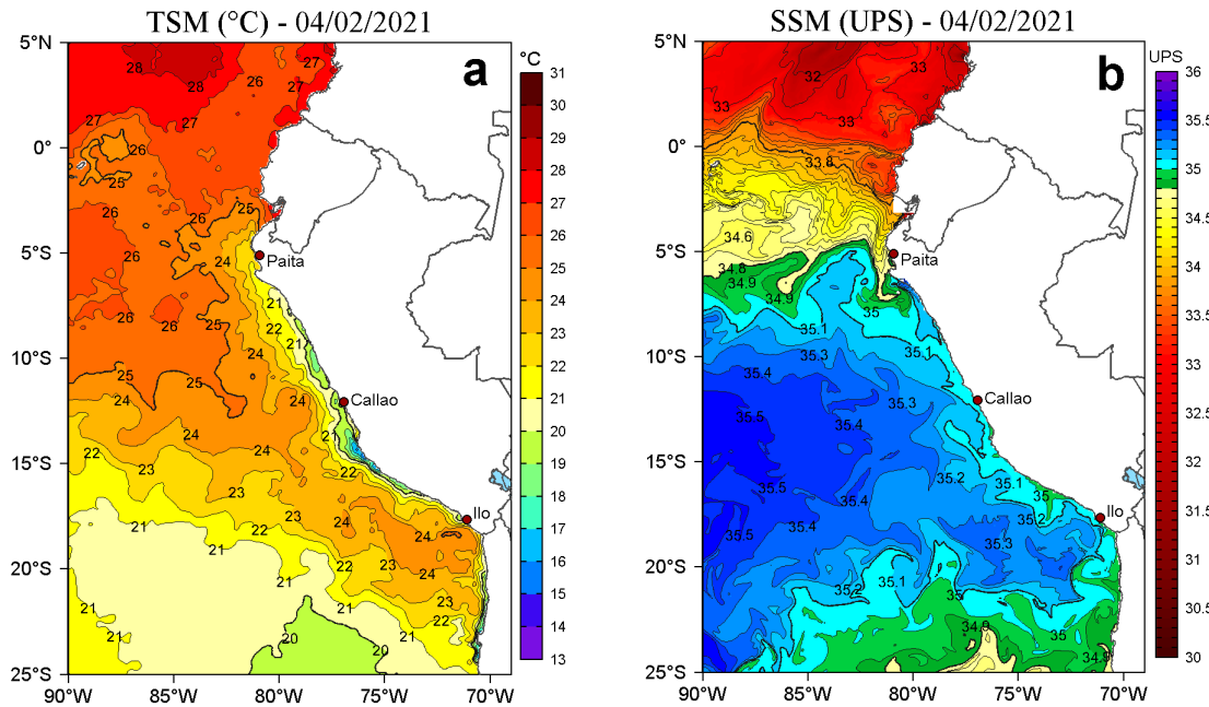
Figura 2. a) Temperatura superficial del mar (TSM, °C) y b) Salinidad superficial del mar (SSM) para el 04 de febrero de 2021. Datos: OSTIA-UKMO-L4-GLOB-v2.0 (UK Met Office, 2012; Donlon et al, 2012) disponible en https://podaac.jpl.nasa.gov/dataset/OSTIA-UKMO-L4-GLOB-v2.0 para (a) y Hybrid Coordinate Ocean Model v. GOF5 3.1 (HYCOM; Halliwell et al., 1998; 2000; Bleck, 2001) para (b).
