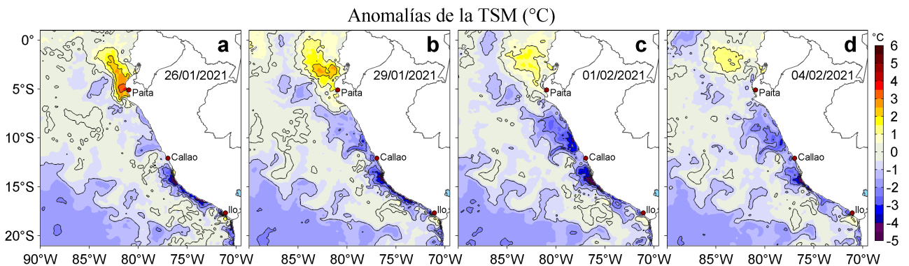
Figura 3. Anomalías de la temperatura superficial del mar (TSM, °C) para los días: a) 26 y b) 29 de enero, c) 01 y d) 04 de febrero de 2021. Las anomalías se calcularon respecto de la climatología para el periodo 2007-2016. Datos: OSTIA-UKMO-L4-GLOB-v2.0 (UK Met Office, 2012; Donlon et al, 2012).
