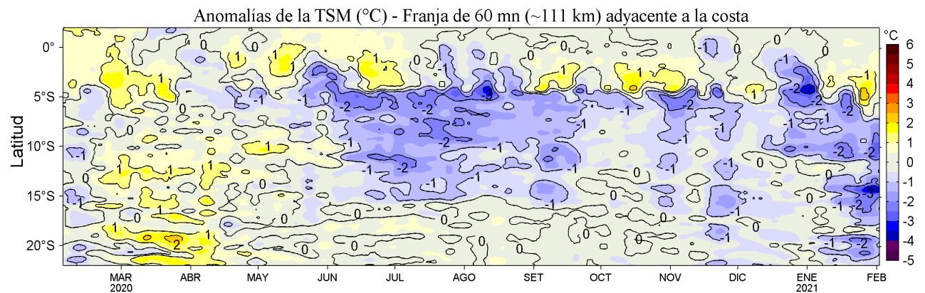
Figura 4. Variación promedio de las anomalías de la temperatura superficial del mar (TSM, °C) para una franja de 60 mn (~111 km) adyacente al litoral peruano para los últimos doce meses al 02 de febrero de 2021. Datos: OSTIA-UKMO-L4-GLOB-v2.0 (UK Met. Office, 2012; Donlon et al, 2012) disponible en https://podaac.jpl.nasa.gov/dataset/OSTIA-UKMO-L4-GLOB-v2.0 . Las anomalías se calcularon con respecto al periodo 2007-2016.
