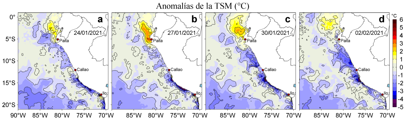
Figura 3. Anomalías de la temperatura superficial del mar (TSM, °C) para los días: a) 24, b) 27 y c) 30 de enero y d) 02 de febrero de 2021. Las anomalías se calcularon respecto de la climatología para el periodo 2007-2016. Datos: OSTIA-UKMO-L4-GLOB-v2.0 (UK Met Office, 2012; Donlon et al, 2012).
