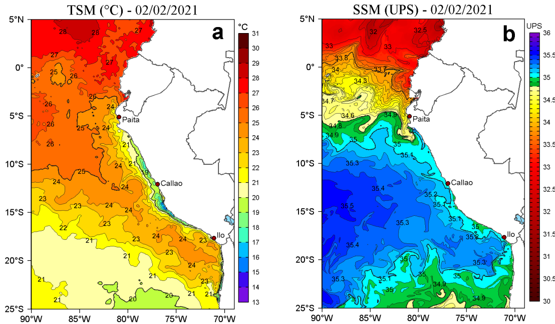
Figura 2. a) Temperatura superficial del mar (TSM, °C) y b) Salinidad superficial del mar (SSM) para el 02 de febrero de 2021. Datos: OSTIA-UKMO-L4-GLOB-v2.0 (UK Met Office, 2012; Donlon et al, 2012) disponible en https://podaac.jpl.nasa.gov/dataset/OSTIA-UKMO-L4-GLOB-v2.0 para (a) y Hybrid Coordinate Ocean Model v. GOFS 3.1 (HYCOM; Halliwell et al., 1998; 2000; Bleck, 2001) para (b).
