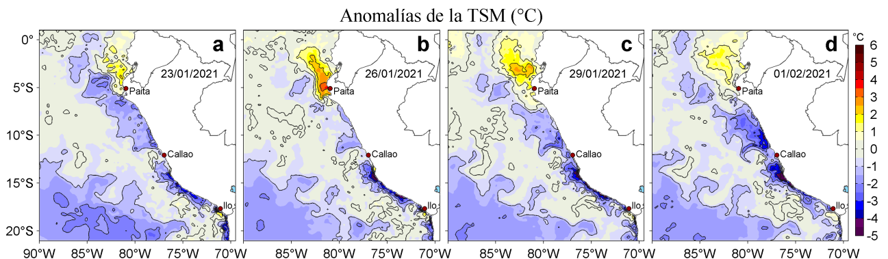
Figura 3. Anomalías de la temperatura superficial del mar (TSM, °C) para los días: a) 23, b) 26 y c) 29 de enero y d) 01 de febrero de 2021. Las anomalías se calcularon respecto de la climatología para el periodo 2007-2016. Datos: OSTIA-UKMO-L4-GLOB-v2.0 (UK Met Office, 2012; Donlon et al, 2012).
