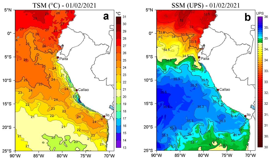
Figura 2. a) Temperatura superficial del mar (TSM, °C) y b) Salinidad superficial del mar (SSM) para el 01 de febrero de 2021. Datos: OSTIA-UKMO-L4-GLOB-v2.0 (UK Met Office, 2012; Donlon et al, 2012) disponible en https://podaac.jpl.nasa.gov/dataset/OSTIA-UKMO-L4-GLOB-v2.0 para (a) y Hybrid Coordinate Ocean Model v. GOFS 3.1 (HYCOM; Halliwell et al., 1998; 2000; Bleck, 2001) para (b).
