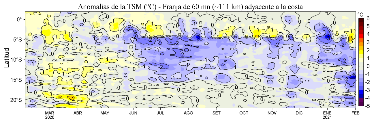
Figura 4. Variación promedio de las anomalías de la temperatura superficial del mar (TSM, °C) para una franja de 60 mn (~111 km) adyacente al litoral peruano para los últimos doce meses al 01 de febrero de 2021. Datos: OSTIA-UKMO-L4-GLOB-v2.0 (UK Met. Office, 2012; Donlon et al, 2012) disponible en https://podaac.jpl.nasa.gov/dataset/OSTIA-UKMO-L4-GLOB-v2.0 . Las anomalías se calcularon con respecto al periodo 2007-2016.
