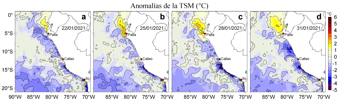
Figura 3. Anomalías de la temperatura superficial del mar (TSM, °C) para los días: a) 22, b) 25, c) 28 y d) 31 de enero de 2021. Las anomalías se calcularon respecto de la climatología para el periodo 2007-2016. Datos: OSTIA-UKMO-L4-GLOB-v2.0 (UK Met Office, 2012; Donlon et al, 2012).
