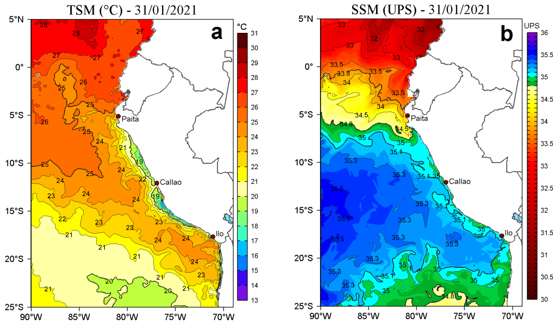
Figura 2. a) Temperatura superficial del mar (TSM, °C) y b) Salinidad superficial del mar (SSM) para el 31 de enero de 2021. Datos: OSTIA-UKMO-L4-GLOB-v2.0 (UK Met Office, 2012; Donlon et al, 2012) disponible en https://podaac.jpl.nasa.gov/dataset/OSTIA-UKMO-L4-GLOB-v2.0 para (a) y Hybrid Coordinate Ocean Model v. GOF5 3.1 (HYCOM; Halliwell et al., 1998; 2000; Bleck, 2001) para (b).
