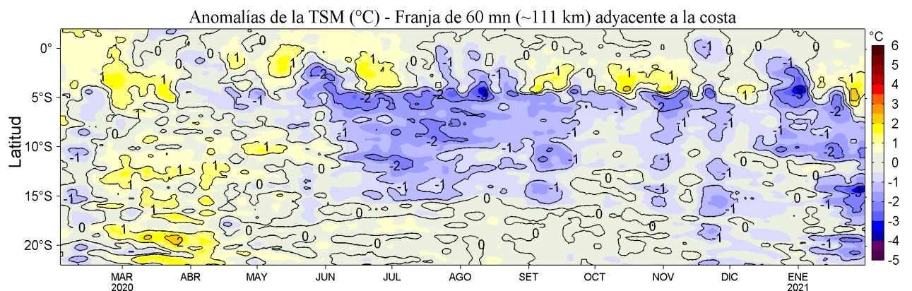
Figura 4. Variación promedio de las anomalías de la temperatura superficial del mar (TSM, °C) para una franja de 60 mn (~111 km) adyacente al litoral peruano para los últimos doce meses al 31 de enero de 2021. Datos: OSTIA-UKMO-L4-GLOB-v2.0 (UK Met. Office, 2012; Donlon et al, 2012) disponible en https://podaac.jpl.nasa.gov/dataset/OSTIA-UKMO-L4-GLOB-v2.0 . Las anomalías se calcularon con respecto al periodo 2007-2016.
