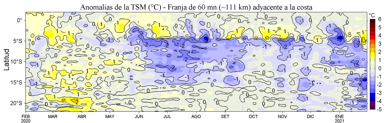
Figura 4. Variación promedio de las anomalías de la temperatura superficial del mar (TSM, °C) para una franja de 60 mn (~111 km) adyacente al litoral peruano para los últimos doce meses al 30 de enero de 2021. Datos: OSTIA-UKMO-L4-GLOB-v2.0 (UK Met. Office, 2012; Donlon et al, 2012) disponible en https://podaac.jpl.nasa.gov/dataset/OSTIA-UKMO-L4-GLOB-v2.0 . Las anomalías se calcularon con respecto al periodo 2007-2016.
