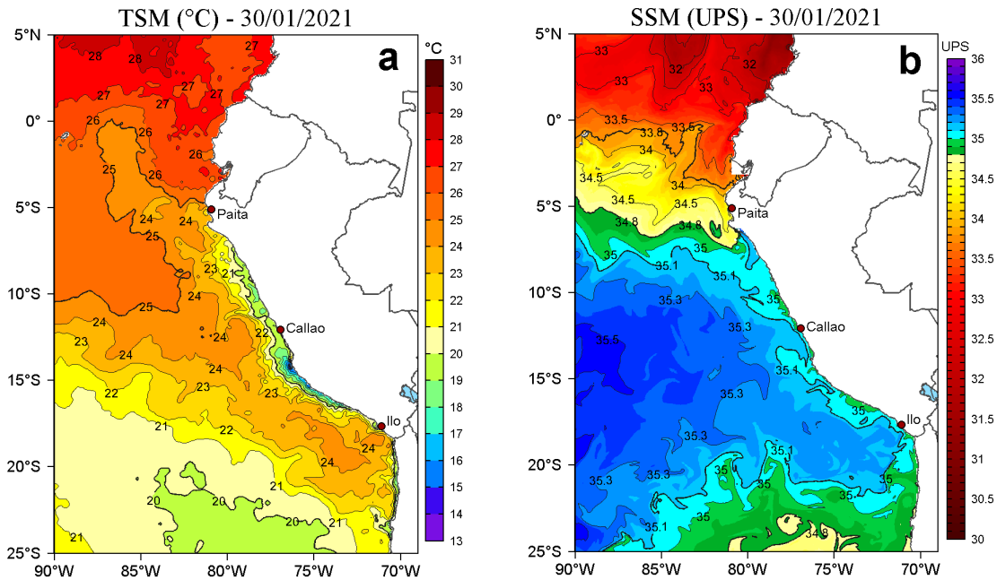
Figura 2. a) Temperatura superficial del mar (TSM, °C) y b) Salinidad superficial del mar (SSM) para el 30 de enero de 2021. Datos: OSTIA-UKMO-L4-GLOB-v2.0 (UK Met Office, 2012; Donlon et al, 2012) disponible en https://podaac.jpl.nasa.gov/dataset/OSTIA-UKMO-L4-GLOB-v2.0 para (a) y Hybrid Coordinate Ocean Model v. GOF5 3.1 (HYCOM; Halliwell et al., 1998; 2000; Bleck, 2001) para (b).
