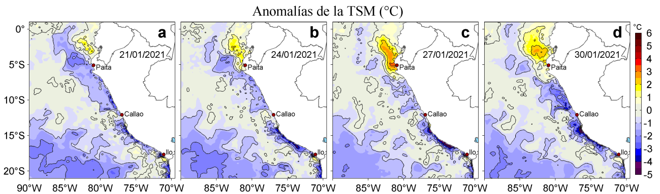
Figura 3. Anomalías de la temperatura superficial del mar (TSM, °C) para los días: a) 21, b) 24, c) 27 y d) 30 de enero de 2021. Las anomalías se calcularon respecto de la climatología para el periodo 2007-2016. Datos: OSTIA-UKMO-L4-GLOB-v2.0 (UK Met Office, 2012; Donlon et al, 2012).
