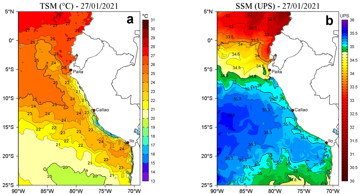
Figura 2. a) Temperatura superficial del mar (TSM, °C) y b) Salinidad superficial del mar (SSM) para el 27 de enero de 2021. Datos: OSTIA-UKMO-L4-GLOB-v2.0 (UK Met Office, 2012; Donlon et al, 2012) disponible en https://podaac.jpl.nasa.gov/dataset/OSTIA-UKMO-L4-GLOB-v2.0 para (a) y Hybrid Coordinate Ocean Model v. GOF3 3.1 (HYCOM; Halliwell et al., 1998; 2000; Bleck, 2001) para (b).
