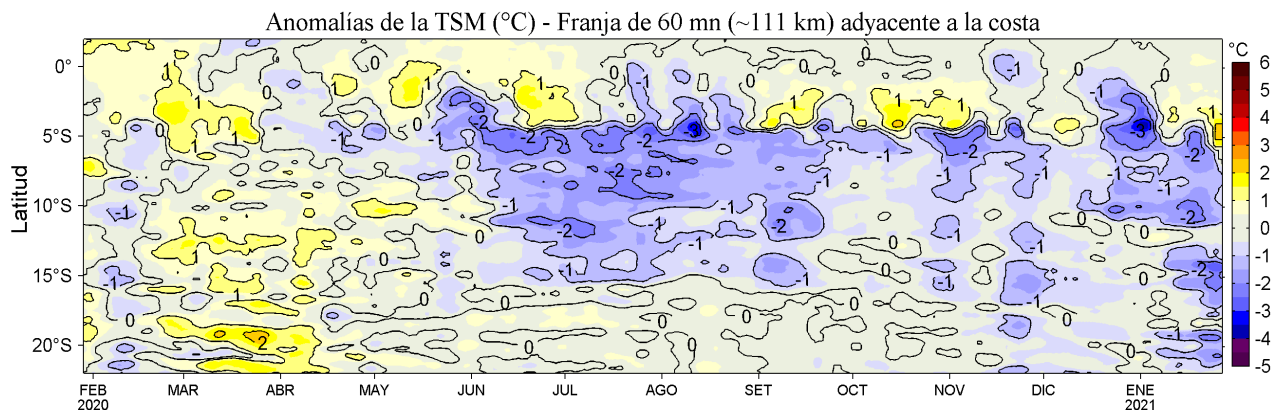
Figura 4. Variación promedio de las anomalías de la temperatura superficial del mar (TSM, °C) para una franja de 60 mn (~111 km) adyacente al litoral peruano para los últimos doce meses al 27 de enero de 2021. Datos: OSTIA-UKMO-L4-GLOB-v2.0 (UK Met. Office, 2012; Donlon et al, 2012) disponible en https://podaac.jpl.nasa.gov/dataset/OSTIA-UKMO-L4-GLOB-v2.0 . Las anomalías se calcularon con respecto al periodo 2007-2016.
