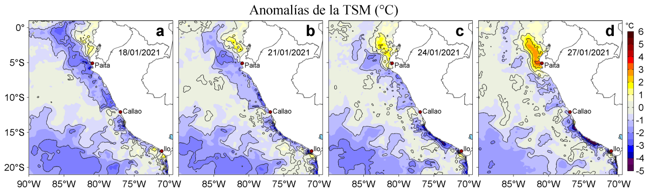
Figura 3. Anomalías de la temperatura superficial del mar (TSM, °C) para los días: a) 18, b) 21, c) 24 y d) 27 de enero de 2021. Las anomalías se calcularon respecto de la climatología para el periodo 2007-2016. Datos: OSTIA-UKMO-L4-GLOB-v2.0 (UK Met Office, 2012; Donlon et al, 2012).
