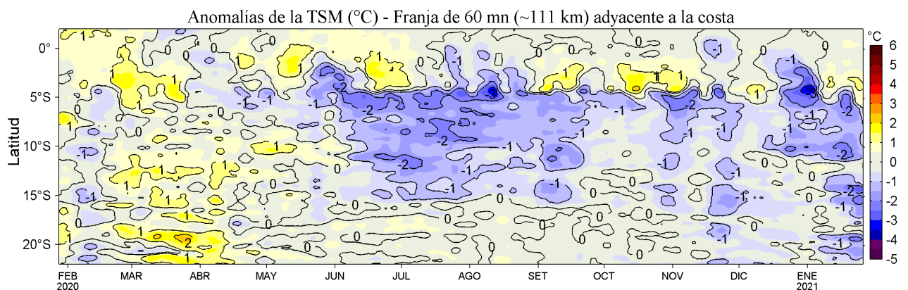
Figura 4. Variación promedio de las anomalías de la temperatura superficial del mar (TSM, °C) para una franja de 60 mn (~111 km) adyacente al litoral peruano para los últimos doce meses al 26 de enero de 2021. Datos: OSTIA-UKMO-L4-GLOB-v2.0 (UK Met. Office, 2012; Donlon et al, 2012) disponible en https://podaac.jpl.nasa.gov/dataset/OSTIA-UKMO-L4-GLOB-v2.0 . Las anomalías se calcularon con respecto al periodo 2007-2016.
