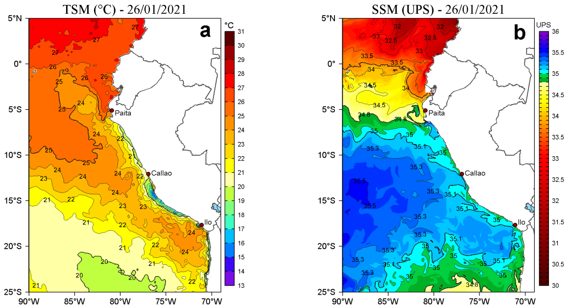
Figura 2. a) Temperatura superficial del mar (TSM, °C) y b) Salinidad superficial del mar (SSM) para el 26 de enero de 2021. Datos: OSTIA-UKMO-L4-GLOB-v2.0 (UK Met Office, 2012; Donlon et al, 2012) disponible en https://podaac.jpl.nasa.gov/dataset/OSTIA-UKMO-L4-GLOB-v2.0 para (a) y Hybrid Coordinate Ocean Model v. GOF3 3.1 (HYCOM; Halliwell et al., 1998; 2000; Bleck, 2001) para (b).
