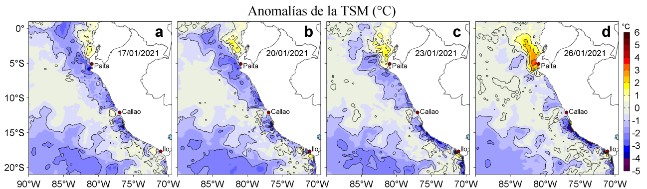
Figura 3. Anomalías de la temperatura superficial del mar (TSM, °C) para los días: a) 17, b) 20, c) 23 y d) 26 de enero de 2021. Las anomalías se calcularon respecto de la climatología para el periodo 2007-2016. Datos: OSTIA-UKMO-L4-GLOB-v2.0 (UK Met Office, 2012; Donlon et al, 2012).
