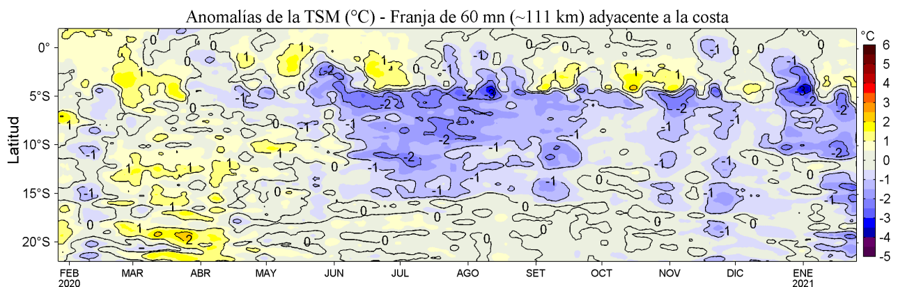
Figura 4. Variación promedio de las anomalías de la temperatura superficial del mar (TSM, °C) para una franja de 60 mn (~111 km) adyacente al litoral peruano para los últimos doce meses al 25 de enero de 2021. Datos: OSTIA-UKMO-L4-GLOB-v2.0 (UK Met. Office, 2012; Donlon et al, 2012) disponible en https://podaac.jpl.nasa.gov/dataset/OSTIA-UKMO-L4-GLOB-v2.0 . Las anomalías se calcularon con respecto al periodo 2007-2016.
