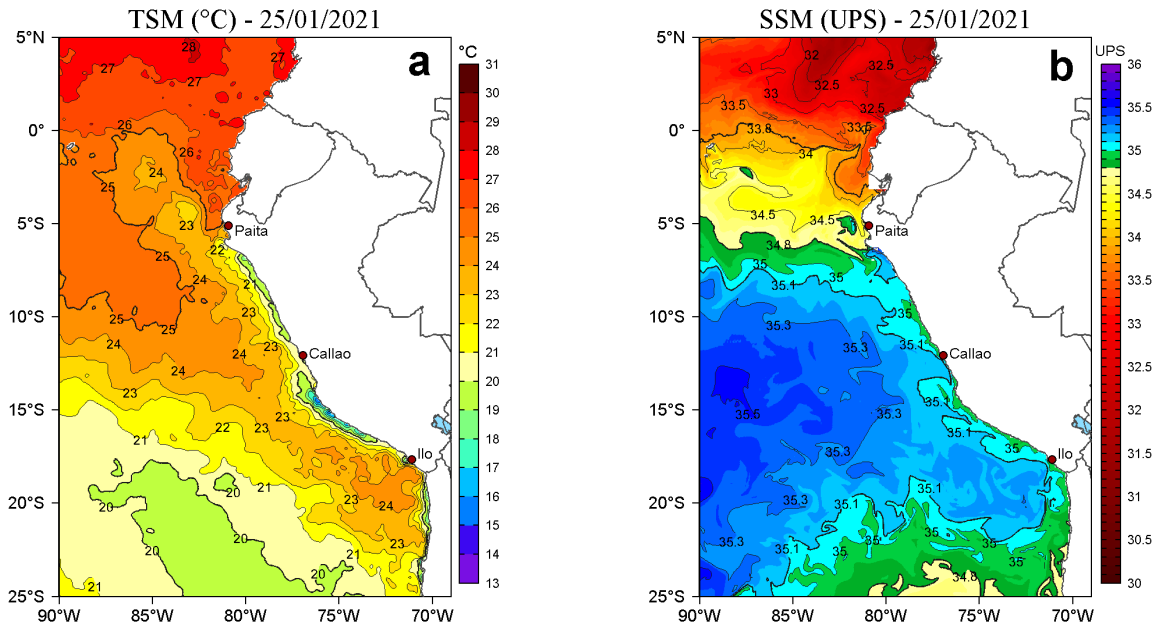
Figura 2. a) Temperatura superficial del mar (TSM, °C) y b) Salinidad superficial del mar (SSM) para el 25 de enero de 2021. Datos: OSTIA-UKMO-L4-GLOB-v2.0 (UK Met Office, 2012; Donlon et al, 2012) disponible en https://podaac.jpl.nasa.gov/dataset/OSTIA-UKMO-L4-GLOB-v2.0 para (a) y Hybrid Coordinate Ocean Model v. GOF3 3.1 (HYCOM; Halliwell et al., 1998; 2000; Bleck, 2001) para (b).
