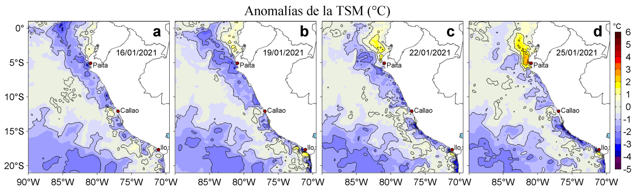
Figura 3. Anomalías de la temperatura superficial del mar (TSM, °C) para los días: a) 16, b) 19, c) 22 y d) 25 de enero de 2021. Las anomalías se calcularon respecto de la climatología para el periodo 2007-2016. Datos: OSTIA-UKMO-L4-GLOB-v2.0 (UK Met Office, 2012; Donlon et al, 2012).
