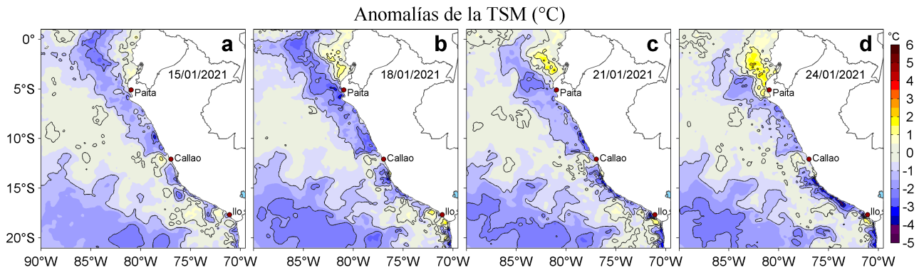
Figura 3. Anomalías de la temperatura superficial del mar (TSM, °C) para los días: a) 15, b) 18, c) 21 y d) 24 de enero de 2021. Las anomalías se calcularon respecto de la climatología para el periodo 2007-2016. Datos: OSTIA-UKMO-L4-GLOB-v2.0 (UK Met Office, 2012; Donlon et al, 2012).
