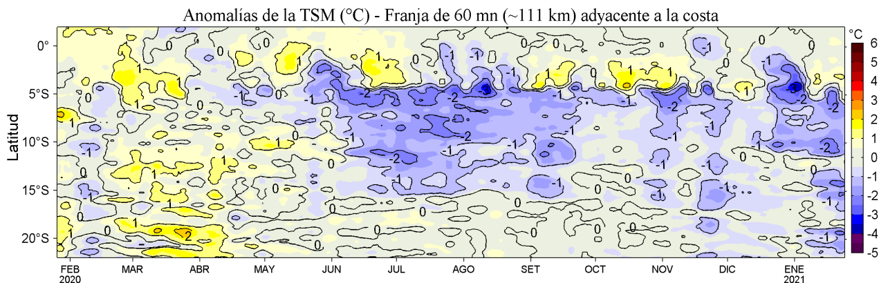
Figura 4. Variación promedio de las anomalías de la temperatura superficial del mar (TSM, °C) para una franja de 60 mn (~111 km) adyacente al litoral peruano para los últimos doce meses al 24 de enero de 2021. Datos: OSTIA-UKMO-L4-GLOB-v2.0 (UK Met. Office, 2012; Donlon et al, 2012) disponible en https://podaac.jpl.nasa.gov/dataset/OSTIA-UKMO-L4-GLOB-v2.0 . Las anomalías se calcularon con respecto al periodo 2007-2016.
