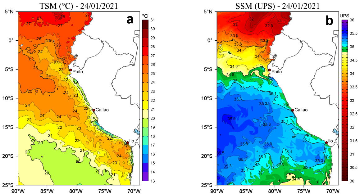
Figura 2. a) Temperatura superficial del mar (TSM, °C) y b) Salinidad superficial del mar (SSM) para el 24 de enero de 2021. Datos: OSTIA-UKMO-L4-GLOB-v2.0 (UK Met Office, 2012; Donlon et al, 2012) disponible en https://podaac.jpl.nasa.gov/dataset/OSTIA-UKMO-L4-GLOB-v2.0 para (a) y Hybrid Coordinate Ocean Model v. GOF3 3.1 (HYCOM; Halliwell et al., 1998; 2000; Bleck, 2001) para (b).
