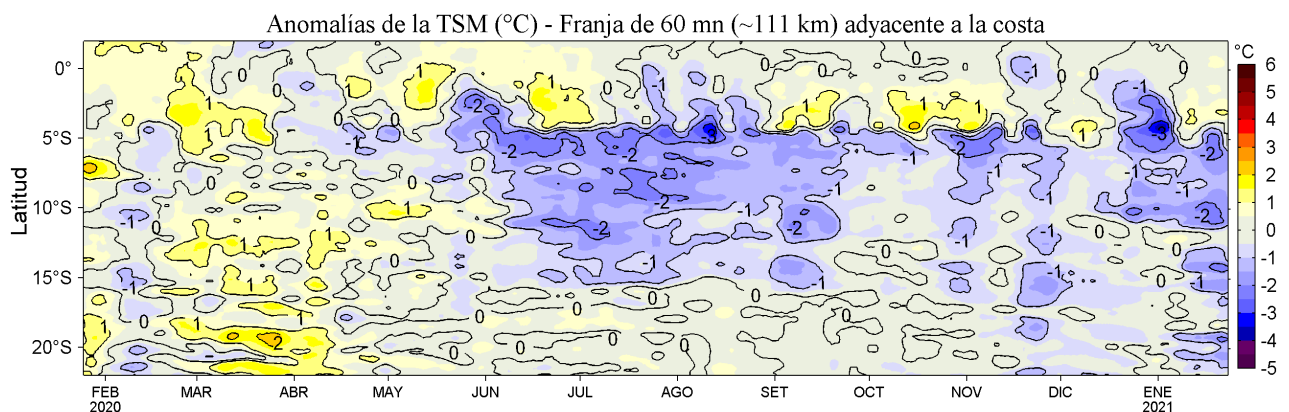
Figura 4. Variación promedio de las anomalías de la temperatura superficial del mar (TSM, °C) para una franja de 60 mn (~111 km) adyacente al litoral peruano para los últimos doce meses al 23 de enero de 2021. Datos: OSTIA-UKMO-L4-GLOB-v2.0 (UK Met. Office, 2012; Donlon et al, 2012) disponible en https://podaac.jpl.nasa.gov/dataset/OSTIA-UKMO-L4-GLOB-v2.0 . Las anomalías se calcularon con respecto al periodo 2007-2016.
