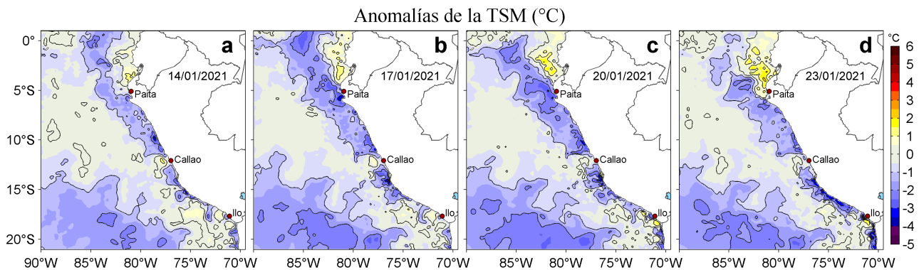
Figura 3. Anomalías de la temperatura superficial del mar (TSM, °C) para los días: a) 14, b) 17, c) 20 y d) 23 de enero de 2021. Las anomalías se calcularon respecto de la climatología para el periodo 2007-2016. Datos: OSTIA-UKMO-L4-GLOB-v2.0 (UK Met Office, 2012; Donlon et al, 2012).
