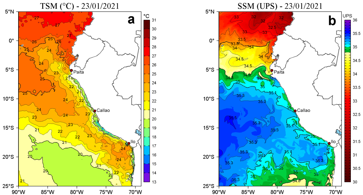
Figura 2. a) Temperatura superficial del mar (TSM, °C) y b) Salinidad superficial del mar (SSM) para el 23 de enero de 2021. Datos: OSTIA-UKMO-L4-GLOB-v2.0 (UK Met Office, 2012; Donlon et al, 2012) disponible en https://podaac.jpl.nasa.gov/dataset/OSTIA-UKMO-L4-GLOB-v2.0 para (a) y Hybrid Coordinate Ocean Model v. GOF3 3.1 (HYCOM; Halliwell et al., 1998; 2000; Bleck, 2001) para (b).
