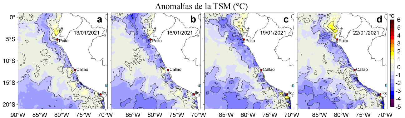
Figura 3. Anomalías de la temperatura superficial del mar (TSM, °C) para los días: a) 13, b) 16, c) 19 y d) 22 de enero de 2021. Las anomalías se calcularon respecto de la climatología para el periodo 2007-2016. Datos: OSTIA-UKMO-L4-GLOB-v2.0 (UK Met Office, 2012; Donlon et al, 2012).
