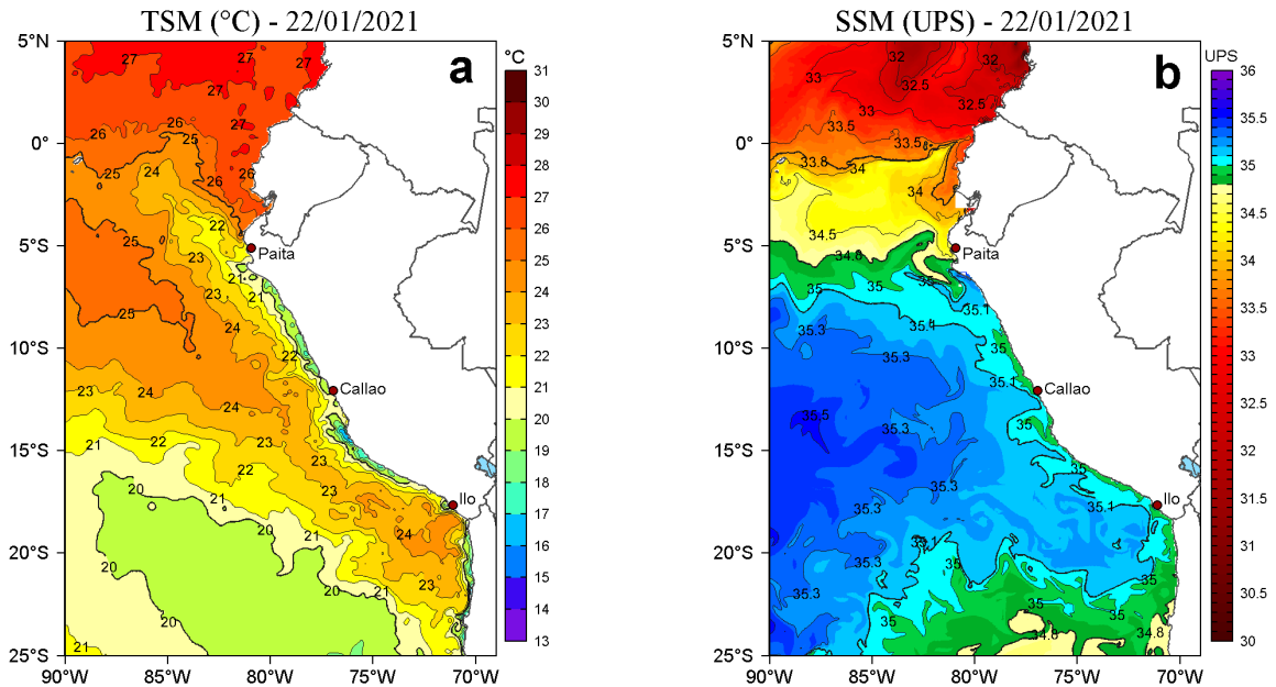
Figura 2. a) Temperatura superficial del mar (TSM, °C) y b) Salinidad superficial del mar (SSM) para el 22 de enero de 2021. Datos: OSTIA-UKMO-L4-GLOB-v2.0 (UK Met Office, 2012; Donlon et al, 2012) disponible en https://podaac.jpl.nasa.gov/dataset/OSTIA-UKMO-L4-GLOB-v2.0 para (a) y Hybrid Coordinate Ocean Model v. GOF3 3.1 (HYCOM; Halliwell et al., 1998; 2000; Bleck, 2001) para (b).
