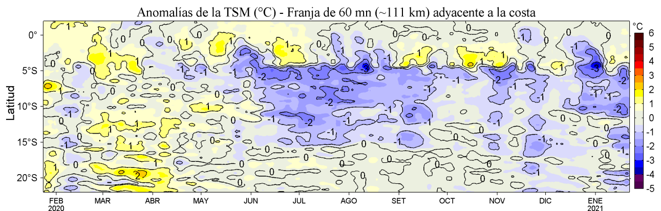
Figura 4. Variación promedio de las anomalías de la temperatura superficial del mar (TSM, °C) para una franja de 60 mn (~111 km) adyacente al litoral peruano para los últimos doce meses al 22 de enero de 2021. Datos: OSTIA-UKMO-L4-GLOB-v2.0 (UK Met. Office, 2012; Donlon et al, 2012) disponible en https://podaac.jpl.nasa.gov/dataset/OSTIA-UKMO-L4-GLOB-v2.0 . Las anomalías se calcularon con respecto al periodo 2007-2016.
