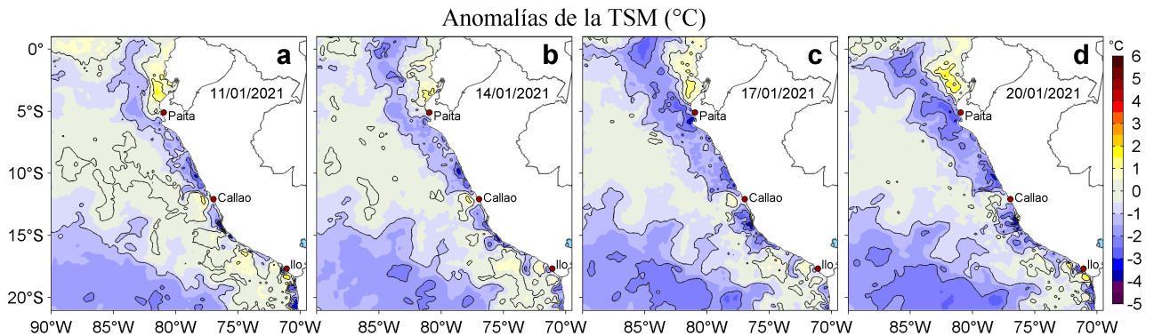
Figura 3. Anomalías de la temperatura superficial del mar (TSM, °C) para los días: a) 11, b) 14, c) 17 y d) 20 de enero de 2021. Las anomalías se calcularon respecto de la climatología para el periodo 2007-2016. Datos: OSTIA-UKMO-L4-GLOB-v2.0 (UK Met Office, 2012; Donlon et al, 2012).
