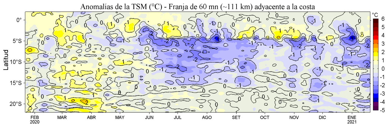
Figura 4. Variación promedio de las anomalías de la temperatura superficial del mar (TSM, °C) para una franja de 60 mn (~111 km) adyacente al litoral peruano para los últimos doce meses al 20 de enero de 2021. Datos: OSTIA-UKMO-L4-GLOB-v2.0 (UK Met. Office, 2012; Donlon et al, 2012) disponible en https://podaac.jpl.nasa.gov/dataset/OSTIA-UKMO-L4-GLOB-v2.0 . Las anomalías se calcularon con respecto al periodo 2007-2016.
