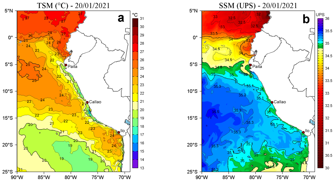
Figura 2. a) Temperatura superficial del mar (TSM, °C) y b) Salinidad superficial del mar (SSM) para el 20 de enero de 2021. Datos: OSTIA-UKMO-L4-GLOB-v2.0 (UK Met Office, 2012; Donlon et al, 2012) disponible en https://podaac.jpl.nasa.gov/dataset/OSTIA-UKMO-L4-GLOB-v2.0 para (a) y Hybrid Coordinate Ocean Model v. GOFS 3.1 (HYCOM; Halliwell et al., 1998; 2000; Bleck, 2001) para (b).
