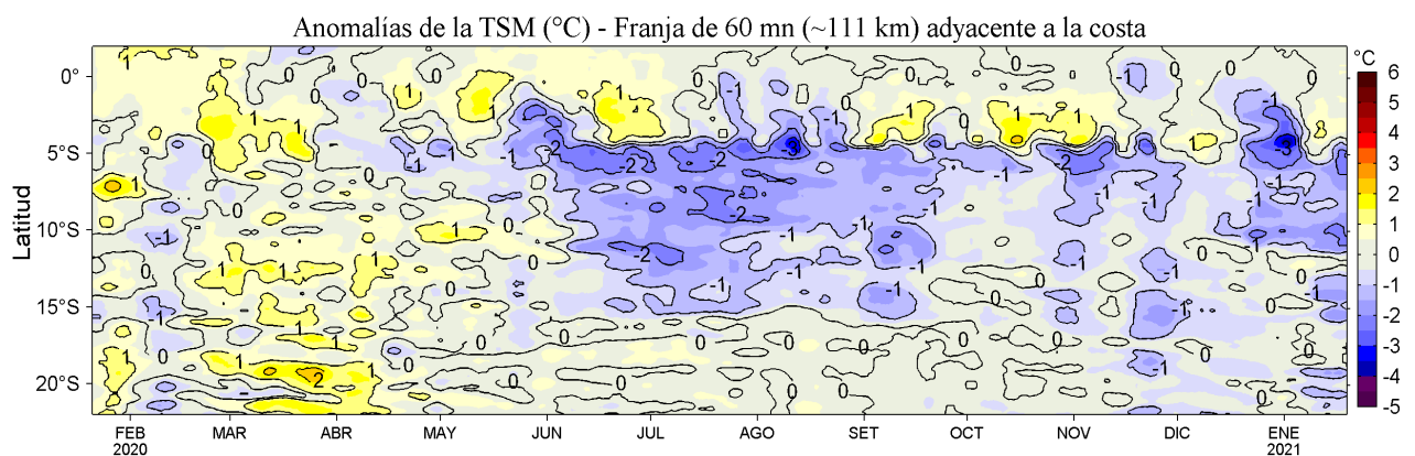
Figura 4. Variación promedio de las anomalías de la temperatura superficial del mar (TSM, °C) para una franja de 60 mn (~111 km) adyacente al litoral peruano para los últimos doce meses al 19 de enero de 2021. Datos: OSTIA-UKMO-L4-GLOB-v2.0 (UK Met. Office, 2012; Donlon et al, 2012) disponible en https://podaac.jpl.nasa.gov/dataset/OSTIA-UKMO-L4-GLOB-v2.0 . Las anomalías se calcularon con respecto al periodo 2007-2016.
