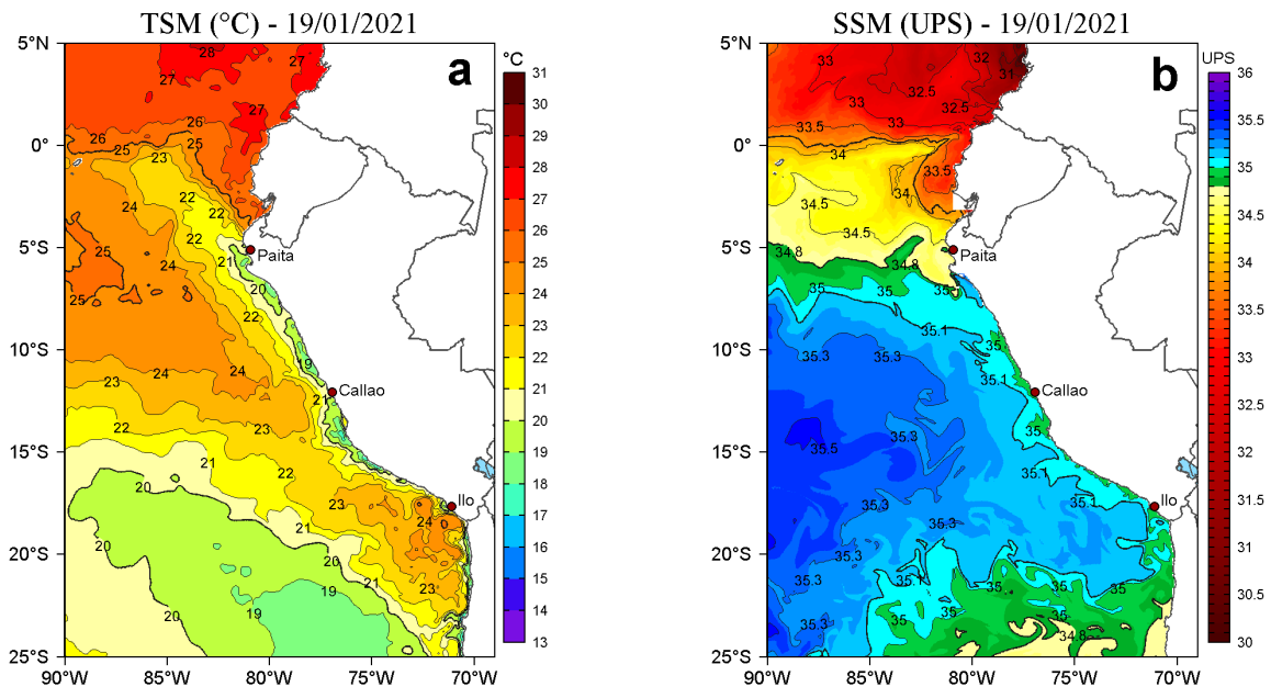
Figura 2. a) Temperatura superficial del mar (TSM, °C) y b) Salinidad superficial del mar (SSM) para el 19 de enero de 2021. Datos: OSTIA-UKMO-L4-GLOB-v2.0 (UK Met Office, 2012; Donlon et al, 2012) disponible en https://podaac.jpl.nasa.gov/dataset/OSTIA-UKMO-L4-GLOB-v2.0 para (a) y Hybrid Coordinate Ocean Model v. GOMS 3.1 (HYCOM; Halliwell et al., 1998; 2000; Bleck, 2001) para (b).
