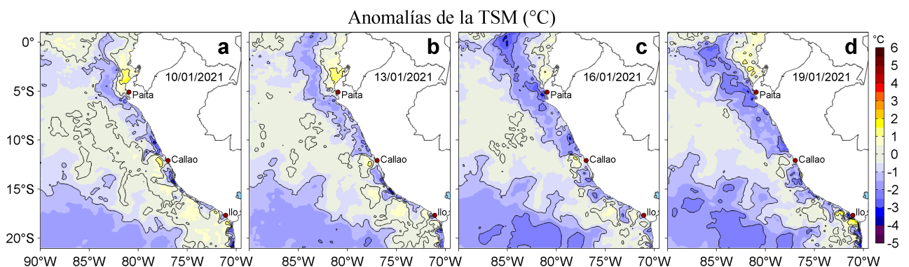
Figura 3. Anomalías de la temperatura superficial del mar (TSM, °C) para los días: a) 10, b) 13, c) 16 y d) 19 de enero de 2021. Las anomalías se calcularon respecto de la climatología para el periodo 2007-2016. Datos: OSTIA-UKMO-L4-GLOB-v2.0 (UK Met Office, 2012; Donlon et al, 2012).
