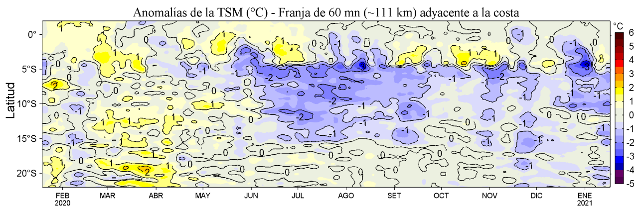
Figura 4. Variación promedio de las anomalías de la temperatura superficial del mar (TSM, °C) para una franja de 60 mn (~111 km) adyacente al litoral peruano para los últimos doce meses al 17 de enero de 2021. Datos: OSTIA-UKMO-L4-GLOB-v2.0 (UK Met. Office, 2012; Donlon et al, 2012) disponible en https://podaac.jpl.nasa.gov/dataset/OSTIA-UKMO-L4-GLOB-v2.0 . Las anomalías se calcularon con respecto al periodo 2007-2016.
