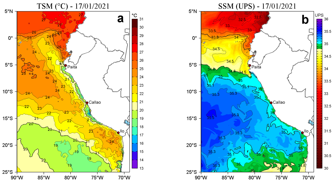
Figura 2. a) Temperatura superficial del mar (TSM, °C) y b) Salinidad superficial del mar (SSM) para el 17 de enero de 2021. Datos: OSTIA-UKMO-L4-GLOB-v2.0 (UK Met Office, 2012; Donlon et al, 2012) disponible en https://podaac.jpl.nasa.gov/dataset/OSTIA-UKMO-L4-GLOB-v2.0 para (a) y Hybrid Coordinate Ocean Model v. GOMS 3.1 (HYCOM; Halliwell et al., 1998; 2000; Bleck, 2001) para (b).
