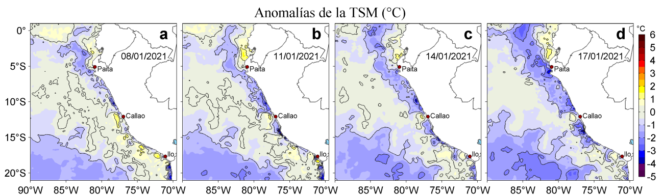
Figura 3. Anomalías de la temperatura superficial del mar (TSM, °C) para los días: a) 08, b) 11, c) 14 y d) 17 de enero de 2021. Las anomalías se calcularon respecto de la climatología para el periodo 2007-2016. Datos: OSTIA-UKMO-L4-GLOB-v2.0 (UK Met Office, 2012; Donlon et al, 2012).
