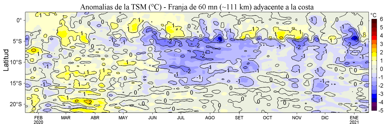
Figura 4. Variación promedio de las anomalías de la temperatura superficial del mar (TSM, °C) para una franja de 60 mn (~111 km) adyacente al litoral peruano para los últimos doce meses al 16 de enero de 2021. Datos: OSTIA-UKMO-L4-GLOB-v2.0 (UK Met. Office, 2012; Donlon et al, 2012) disponible en https://podaac.jpl.nasa.gov/dataset/OSTIA-UKMO-L4-GLOB-v2.0 . Las anomalías se calcularon con respecto al periodo 2007-2016.
