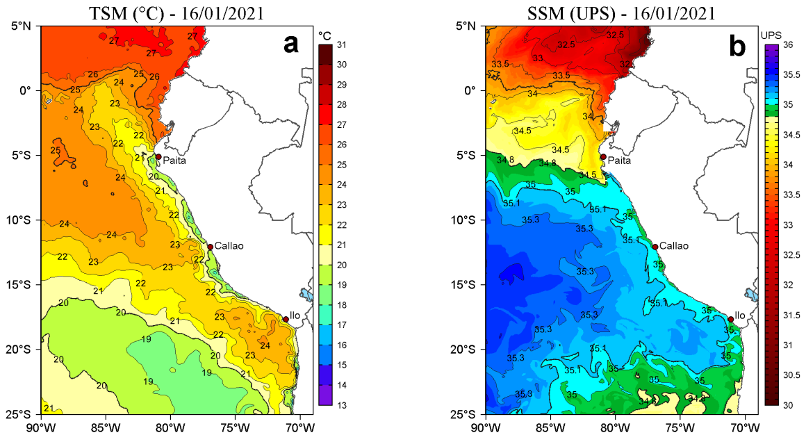
Figura 2. a) Temperatura superficial del mar (TSM, °C) y b) Salinidad superficial del mar (SSM) para el 16 de enero de 2021. Datos: OSTIA-UKMO-L4-GLOB-v2.0 (UK Met Office, 2012; Donlon et al, 2012) disponible en https://podaac.jpl.nasa.gov/dataset/OSTIA-UKMO-L4-GLOB-v2.0 para (a) y Hybrid Coordinate Ocean Model v. GOMS 3.1 (HYCOM; Halliwell et al., 1998; 2000; Bleck, 2001) para (b).
