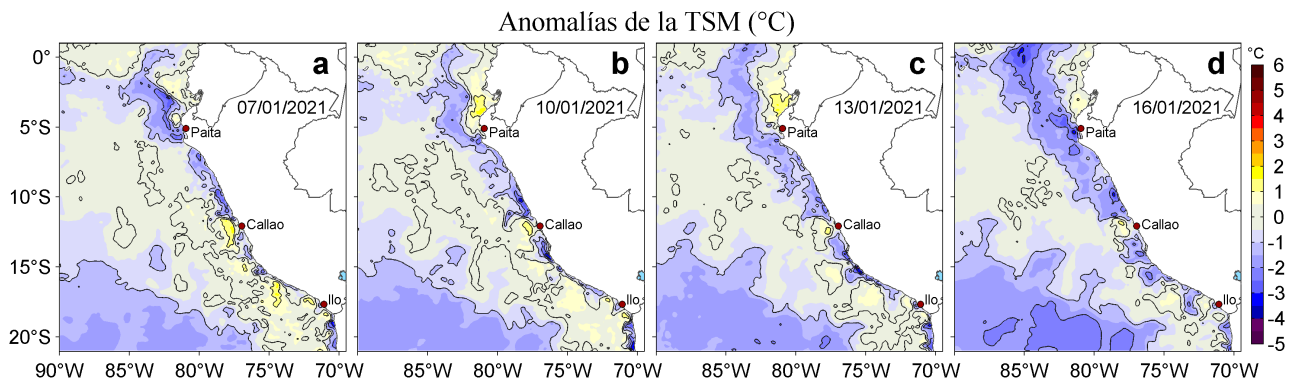
Figura 3. Anomalías de la temperatura superficial del mar (TSM, °C) para los días: a) 07, b) 10, c) 13 y d) 16 de enero de 2021. Las anomalías se calcularon respecto de la climatología para el periodo 2007-2016. Datos: OSTIA-UKMO-L4-GLOB-v2.0 (UK Met Office, 2012; Donlon et al, 2012).
