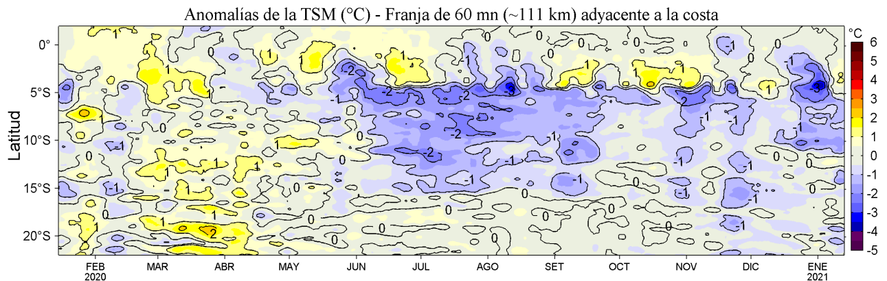
Figura 4. Variación promedio de las anomalías de la temperatura superficial del mar (TSM, °C) para una franja de 60 mn (~111 km) adyacente al litoral peruano para los últimos doce meses al 13 de enero de 2021. Datos: OSTIA-UKMO-L4-GLOB-v2.0 (UK Met. Office, 2012; Donlon et al, 2012) disponible en https://podaac.jpl.nasa.gov/dataset/OSTIA-UKMO-L4-GLOB-v2.0 . Las anomalías se calcularon con respecto al periodo 2007-2016.
