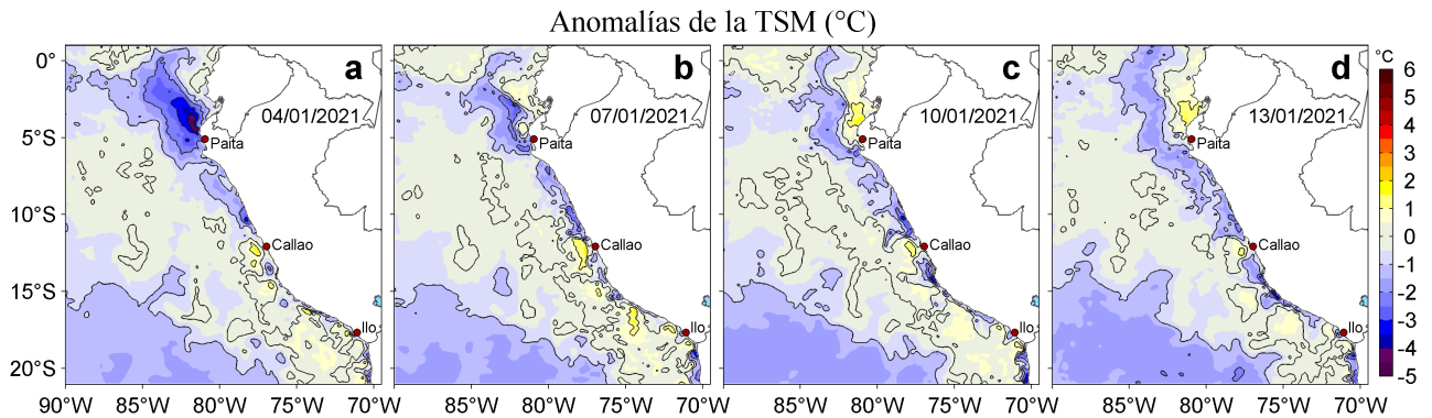
Figura 3. Anomalías de la temperatura superficial del mar (TSM, °C) para los días: a) 04, b) 07, c) 10 y d) 13 de enero de 2021. Las anomalías se calcularon respecto de la climatología para el periodo 2007-2016. Datos: OSTIA-UKMO-L4-GLOB-v2.0 (UK Met Office, 2012; Donlon et al, 2012).
