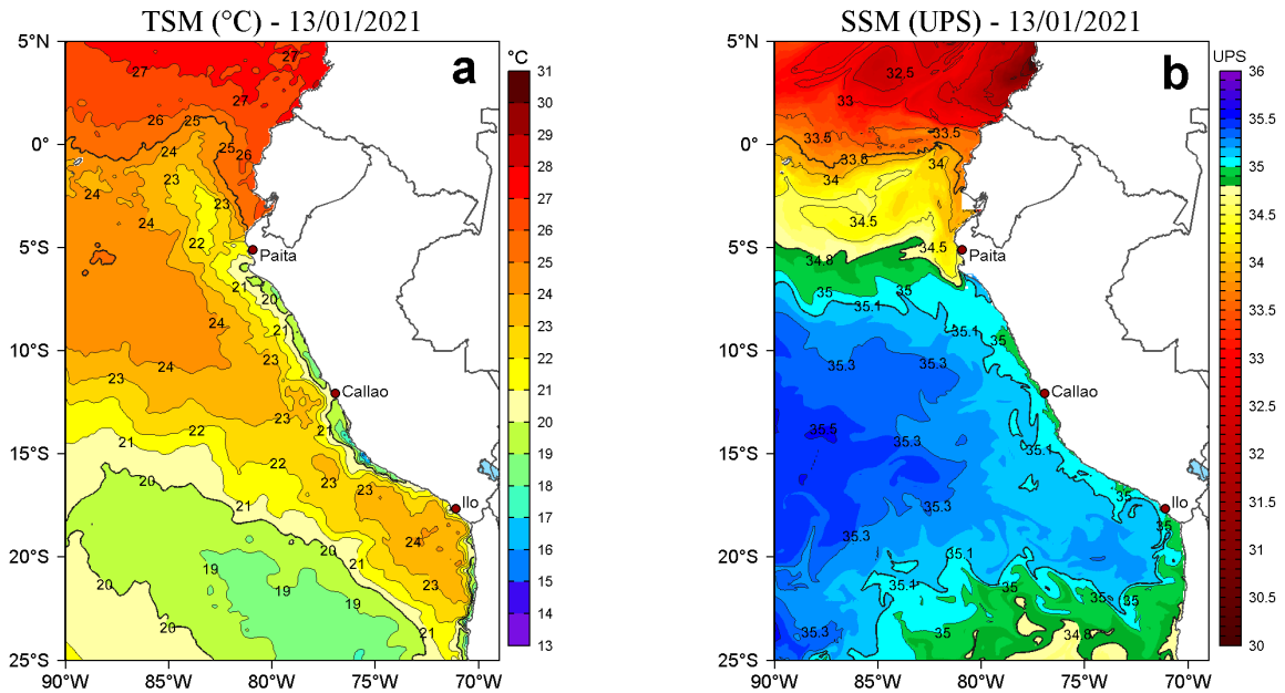
Figura 2. a) Temperatura superficial del mar (TSM, °C) y b) Salinidad superficial del mar (SSM) para el 13 de enero de 2021. Datos: OSTIA-UKMO-L4-GLOB-v2.0 (UK Met Office, 2012; Donlon et al, 2012) disponible en https://podaac.jpl.nasa.gov/dataset/OSTIA-UKMO-L4-GLOB-v2.0 para (a) y Hybrid Coordinate Ocean Model v. GOFS 3.1 (HYCOM; Halliwell et al., 1998; 2000; Bleck, 2001) para (b).
