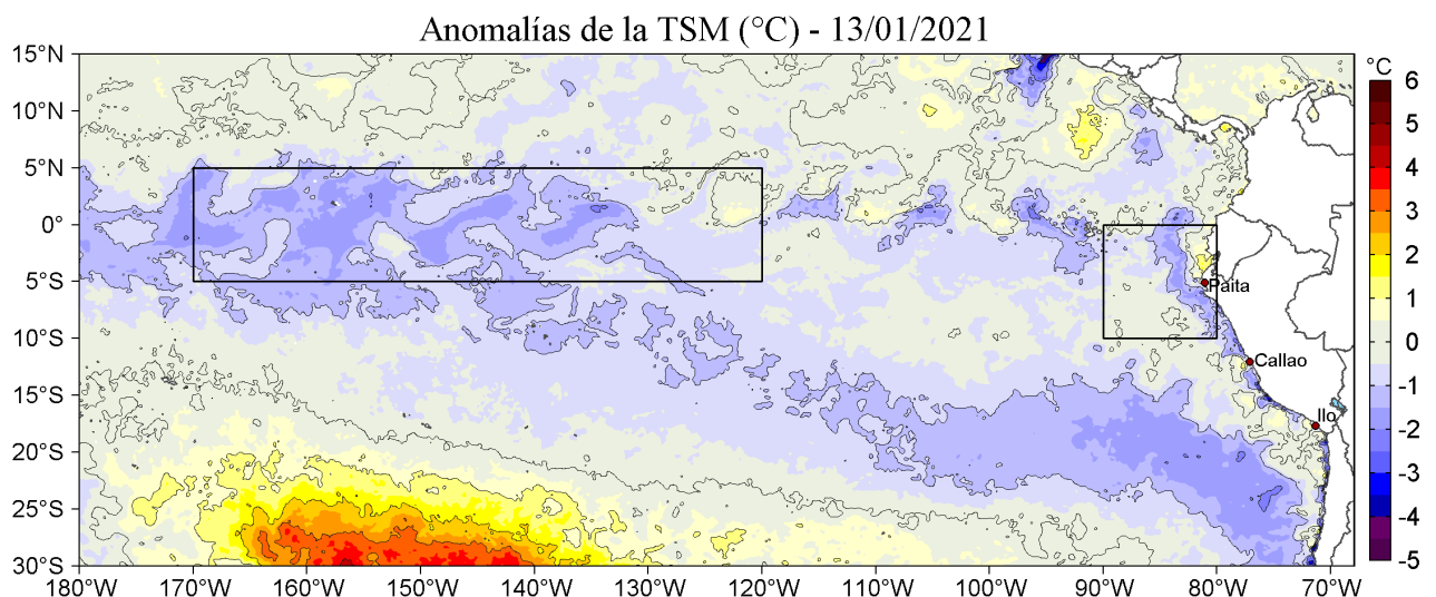
Figura 1. Anomalías de la temperatura superficial del mar (TSM, °C) en el océano Pacífico tropical. Las regiones Niño 3.4 ( 5^{\circ}\text{N} - 5^{\circ}\text{S} , 170^{\circ}\text{W} - 120^{\circ}\text{W} ) y Niño 1+2 ( 0^{\circ} - 10^{\circ}\text{S} , 90^{\circ}\text{W} - 80^{\circ}\text{W} ) en los sectores central y oriental del océano, respectivamente, están delimitadas con una línea de color negro. Las anomalías se estimaron de acuerdo a la climatología para el periodo 2007-2016. Los datos provienen de OSTIA-UKMO-L4-GLOB-v2.0 (UK Met Office, 2012; Donlon et al, 2012) y están disponibles en https://podaac.jpl.nasa.gov/dataset/OSTIA-UKMO-L4-GLOB-v2.0 .
