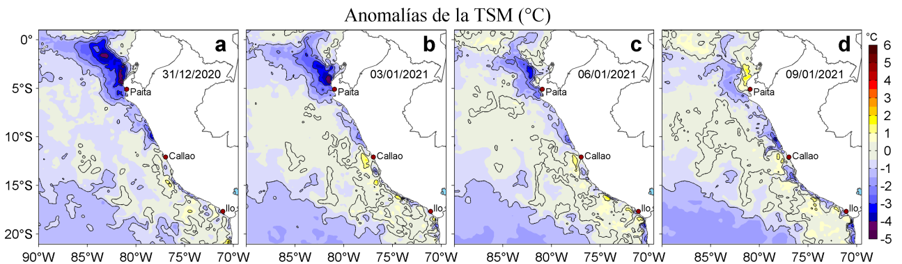
Figura 3. Anomalías de la temperatura superficial del mar (TSM, °C) para los días: a) 31 de diciembre de 2020, b) 03, c) 06 y d) 09 de enero de 2021. Las anomalías se calcularon respecto de la climatología para el periodo 2007-2016. Datos: OSTIA-UKMO-L4-GLOB-v2.0 (UK Met Office, 2012; Donlon et al, 2012).
