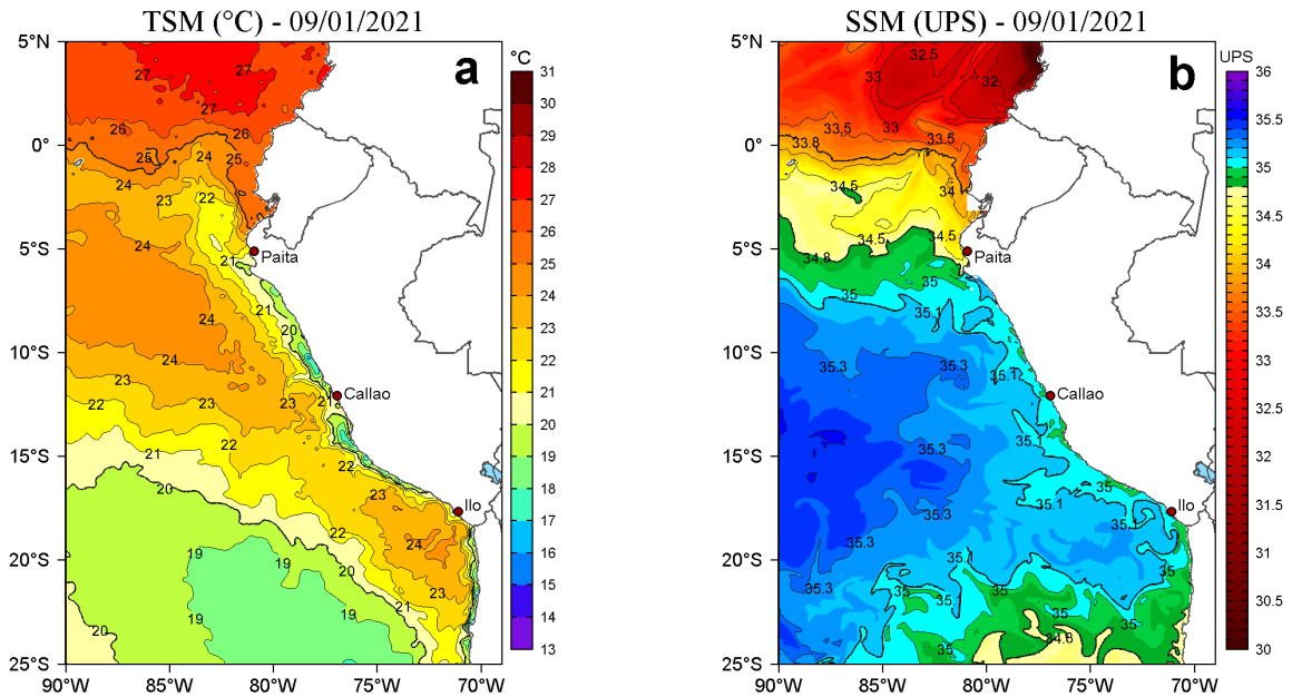
Figura 2. a) Temperatura superficial del mar (TSM, °C) y b) Salinidad superficial del mar (SSM) para el 09 de enero de 2021. Datos: OSTIA-UKMO-L4-GLOB-v2.0 (UK Met Office, 2012; Donlon et al, 2012) disponible en https://podaac.jpl.nasa.gov/dataset/OSTIA-UKMO-L4-GLOB-v2.0 para (a) y Hybrid Coordinate Ocean Model v. GOFS 3.1 (HYCOM; Halliwell et al., 1998; 2000; Bleck, 2001) para (b).
