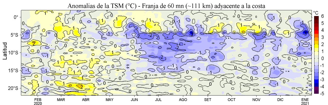
Figura 4. Variación promedio de las anomalías de la temperatura superficial del mar (TSM, °C) para una franja de 60 m.n. (~111 km) adyacente al litoral peruano para los últimos doce meses al 09 de enero de 2021. Datos: OSTIA-UKMO-L4-GLOB-v2.0 (UK Met. Office, 2012; Donlon et al, 2012) disponible en https://podaac.jpl.nasa.gov/dataset/OSTIA-UKMO-L4-GLOB-v2.0 . Las anomalías se calcularon con respecto al periodo 2007-2016.
