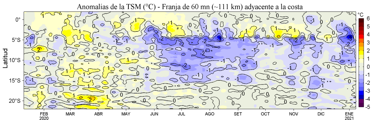
Figura 4. Variación promedio de las anomalías de la temperatura superficial del mar (TSM, °C) para una franja de 60 mn (~111 km) adyacente al litoral peruano para los últimos doce meses al 08 de enero de 2021. Datos: OSTIA-UKMO-L4-GLOB-v2.0 (UK Met. Office, 2012; Donlon et al, 2012) disponible en https://podaac.jpl.nasa.gov/dataset/OSTIA-UKMO-L4-GLOB-v2.0 . Las anomalías se calcularon con respecto al periodo 2007-2016.
