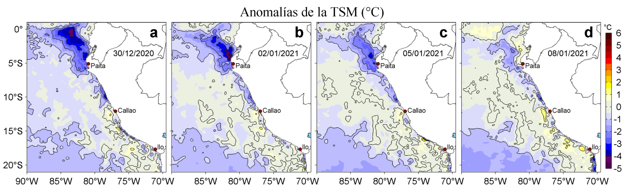
Figura 3. Anomalías de la temperatura superficial del mar (TSM, °C) para los días: a) 30 de diciembre de 2020, b) 02, c) 05 y d) 08 de enero de 2021. Las anomalías se calcularon respecto de la climatología para el periodo 2007-2016. Datos: OSTIA-UKMO-L4-GLOB-v2.0 (UK Met Office, 2012; Donlon et al, 2012).
