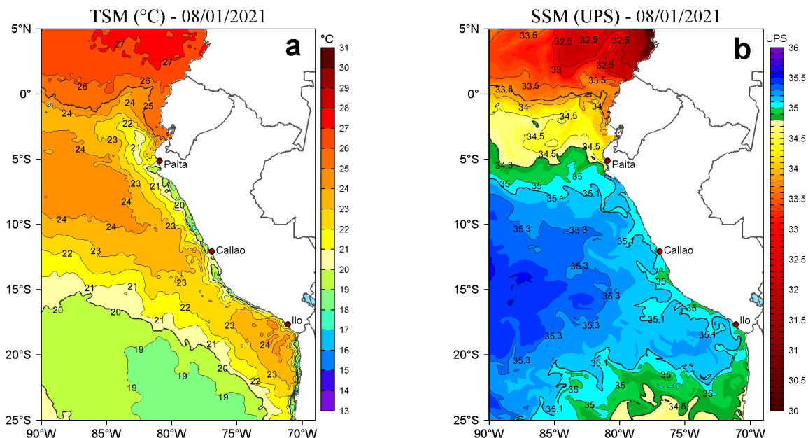
Figura 2. a) Temperatura superficial del mar (TSM, °C) y b) Salinidad superficial del mar (SSM) para el 08 de enero de 2021. Datos: OSTIA-UKMO-L4-GLOB-v2.0 (UK Met Office, 2012; Donlon et al, 2012) disponible en https://podaac.jpl.nasa.gov/dataset/OSTIA-UKMO-L4-GLOB-v2.0 para (a) y Hybrid Coordinate Ocean Model v. GOMS 3.1 (HYCOM; Halliwell et al., 1998; 2000; Bleck, 2001) para (b).
