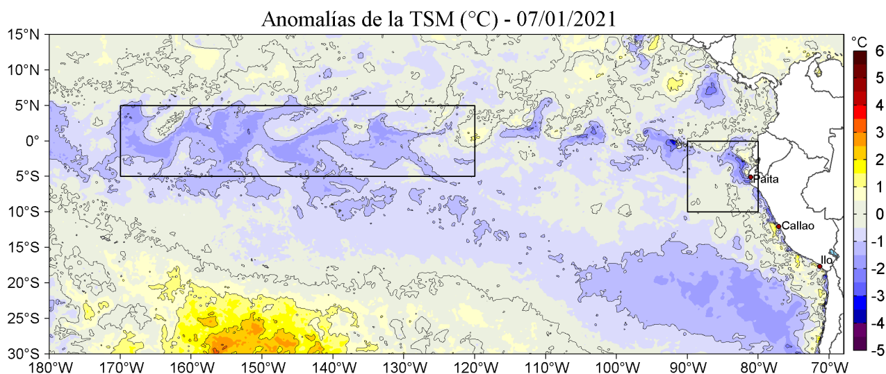
Figura 1. Anomalías de la temperatura superficial del mar (TSM, °C) en el océano Pacífico tropical. Las regiones Niño 3.4 ( 5^{\circ} N - 5^{\circ} S, 170^{\circ} W - 120^{\circ} W) y Niño 1+2 ( 0^{\circ} - 10^{\circ} S, 90^{\circ} W - 80^{\circ} W) en los sectores central y oriental del océano, respectivamente, están delimitadas con una línea de color negro. Las anomalías se estimaron de acuerdo a la climatología para el periodo 2007-2016. Los datos provienen de OSTIA-UKMO-L4-GLOB-v2.0 (UK Met Office, 2012; Donlon et al, 2012) y están disponibles en https://podaac.jpl.nasa.gov/dataset/OSTIA-UKMO-L4-GLOB-v2.0 .
