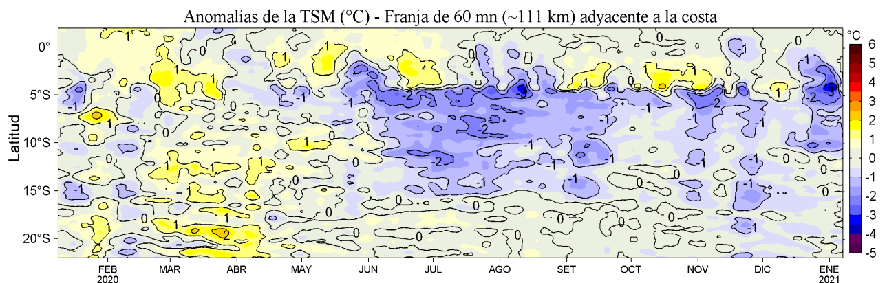
Figura 4. Variación promedio de las anomalías de la temperatura superficial del mar (TSM, °C) para una franja de 60 mn (~111 km) adyacente al litoral peruano para los últimos doce meses al 07 de enero de 2021. Datos: OSTIA-UKMO-L4-GLOB-v2.0 (UK Met. Office, 2012; Donlon et al, 2012) disponible en https://podaac.jpl.nasa.gov/dataset/OSTIA-UKMO-L4-GLOB-v2.0 . Las anomalías se calcularon con respecto al periodo 2007-2016.
