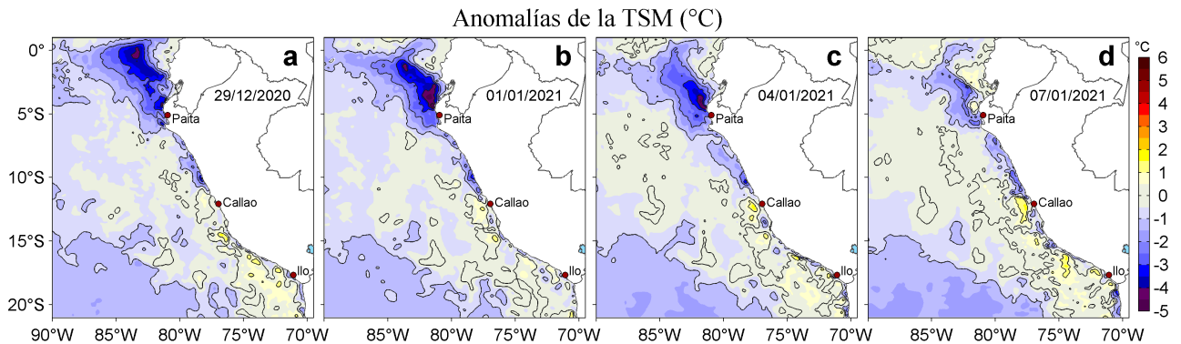
Figura 3. Anomalías de la temperatura superficial del mar (TSM, °C) para los días: a) 29 de diciembre de 2020, b) 01, c) 04 y d) 07 de enero de 2021. Las anomalías se calcularon respecto de la climatología para el periodo 2007-2016. Datos: OSTIA-UKMO-L4-GLOB-v2.0 (UK Met Office, 2012; Donlon et al, 2012).
