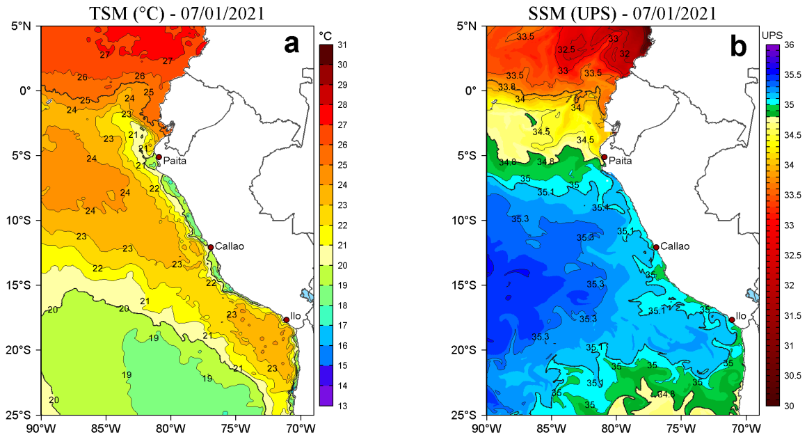
Figura 2. a) Temperatura superficial del mar (TSM, °C) y b) Salinidad superficial del mar (SSM) para el 07 de enero de 2021. Datos: OSTIA-UKMO-L4-GLOB-v2.0 (UK Met Office, 2012; Donlon et al, 2012) disponible en https://podaac.jpl.nasa.gov/dataset/OSTIA-UKMO-L4-GLOB-v2.0 para (a) y Hybrid Coordinate Ocean Model v. GOF3 3.1 (HYCOM; Halliwell et al., 1998; 2000; Bleck, 2001) para (b).
