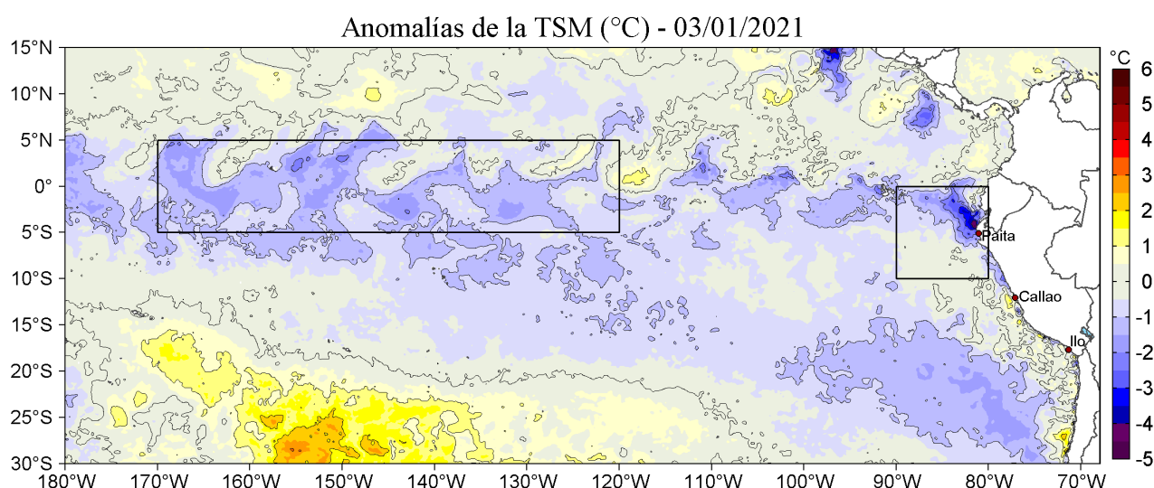
Figura 1. Anomalías de la temperatura superficial del mar (TSM, °C) en el océano Pacífico tropical. Las regiones Niño 3.4 ( 5^{\circ}\text{N} - 5^{\circ}\text{S} , 170^{\circ}\text{W} - 120^{\circ}\text{W} ) y Niño 1+2 ( 0 - 10^{\circ}\text{S} , 90^{\circ}\text{W} - 80^{\circ}\text{W} ) en los sectores central y oriental del océano, respectivamente, están delimitadas con una línea de color negro. Las anomalías se estimaron de acuerdo a la climatología para el periodo 2007-2016. Los datos provienen de OSTIA-UKMO-L4-GLOB-v2.0 (UK Met Office, 2012; Donlon et al, 2012) y están disponibles en https://podaac.jpl.nasa.gov/dataset/OSTIA-UKMO-L4-GLOB-v2.0 .
