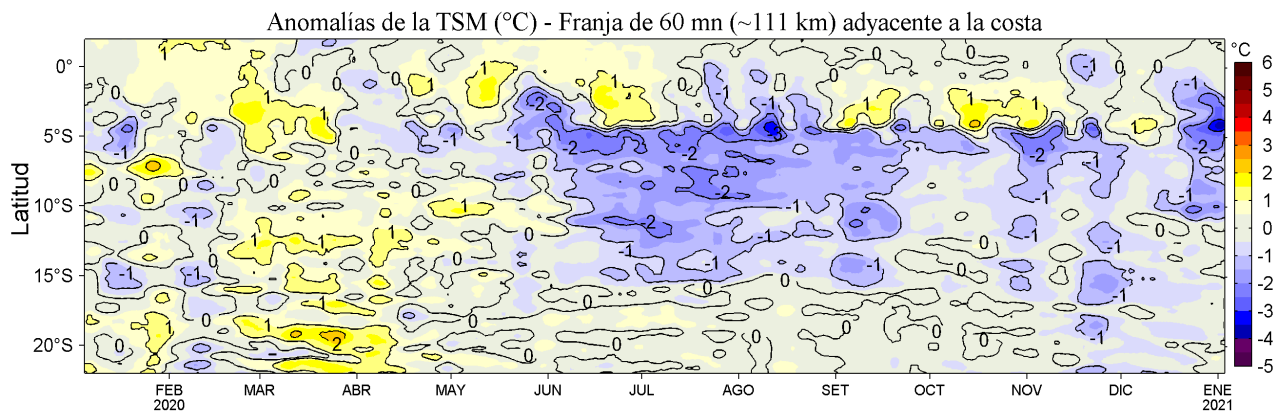
Figura 4. Variación promedio de las anomalías de la temperatura superficial del mar (TSM, °C) para una franja de 60 mn (~111 km) adyacente al litoral peruano para los últimos doce meses al 03 de enero de 2021. Datos: OSTIA-UKMO-L4-GLOB-v2.0 (UK Met. Office, 2012; Donlon et al, 2012) disponible en https://podaac.jpl.nasa.gov/dataset/OSTIA-UKMO-L4-GLOB-v2.0 . Las anomalías se calcularon con respecto al periodo 2007-2016.
