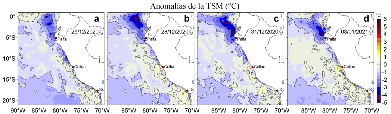
Figura 3. Anomalías de la temperatura superficial del mar (TSM, °C) para los días: a) 25, b) 28 y c) 31 de diciembre de 2020 y d) 03 de enero de 2021. Las anomalías se calcularon respecto de la climatología para el periodo 2007-2016. Datos: OSTIA-UKMO-L4-GLOB-v2.0 (UK Met Office, 2012; Donlon et al, 2012).
