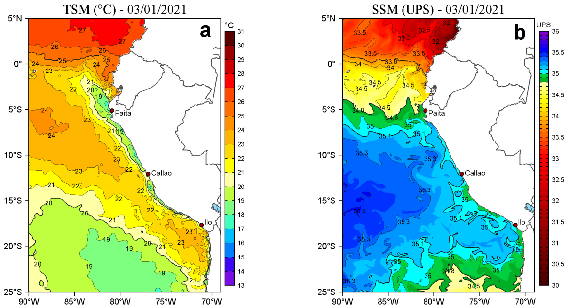
Figura 2. a) Temperatura superficial del mar (TSM, °C) y b) Salinidad superficial del mar (SSM) para el 03 de enero de 2021. Datos: OSTIA-UKMO-L4-GLOB-v2.0 (UK Met Office, 2012; Donlon et al, 2012) disponible en https://podaac.jpl.nasa.gov/dataset/OSTIA-UKMO-L4-GLOB-v2.0 para (a) y Hybrid Coordinate Ocean Model v. GOFS 3.1 (HYCOM; Halliwell et al., 1998; 2000; Bleck, 2001) para (b).
