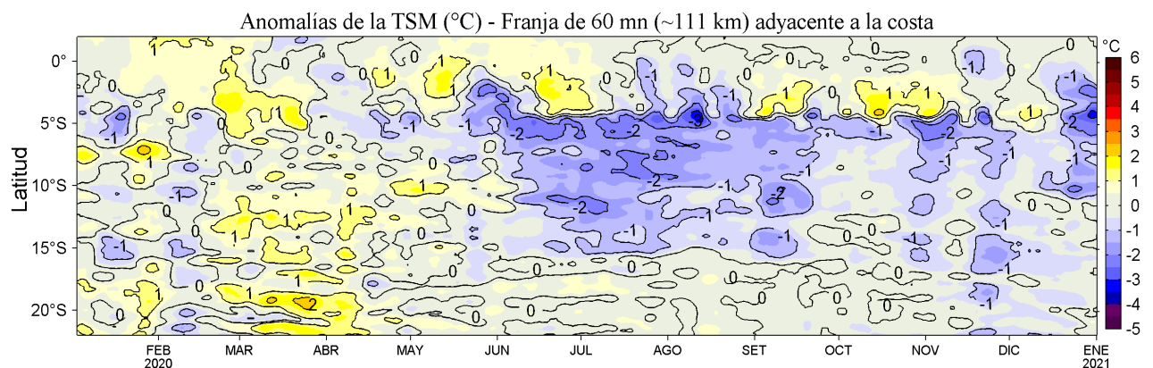
Figura 4. Variación promedio de las anomalías de la temperatura superficial del mar (TSM, °C) para una franja de 60 mn (~111 km) adyacente al litoral peruano para los últimos doce meses al 01 de enero de 2021. Datos: OSTIA-UKMO-L4-GLOB-v2.0 (UK Met. Office, 2012; Donlon et al, 2012) disponible en https://podaac.jpl.nasa.gov/dataset/OSTIA-UKMO-L4-GLOB-v2.0 . Las anomalías se calcularon con respecto al periodo 2007-2016.
