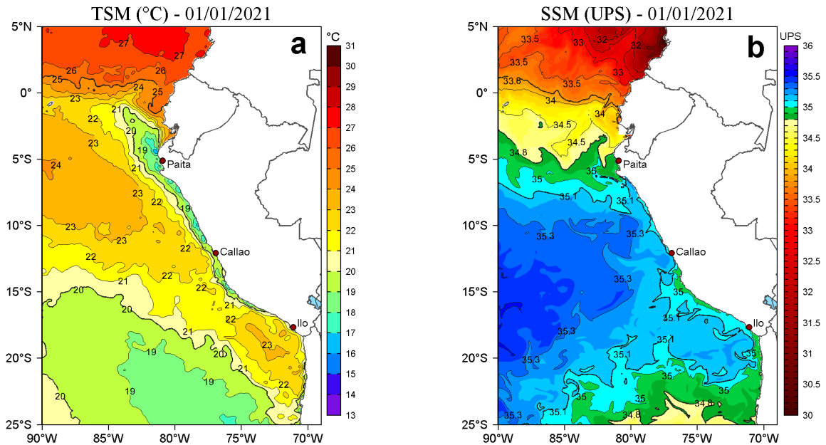
Figura 2. a) Temperatura superficial del mar (TSM, °C) y b) Salinidad superficial del mar (SSM) para el 01 de enero de 2021. Datos: OSTIA-UKMO-L4-GLOB-v2.0 (UK Met Office, 2012; Donlon et al, 2012) disponible en https://podaac.jpl.nasa.gov/dataset/OSTIA-UKMO-L4-GLOB-v2.0 para (a) y Hybrid Coordinate Ocean Model v. GOFS 3.1 (HYCOM; Halliwell et al., 1998; 2000; Bleck, 2001) para (b).
