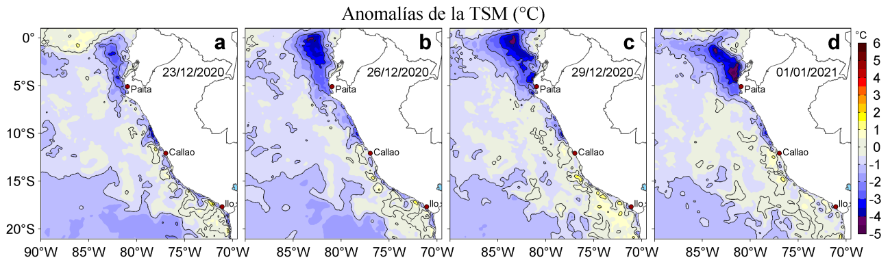
Figura 3. Anomalías de la temperatura superficial del mar (TSM, °C) para los días: a) 23, b) 26 y c) 29 de diciembre de 2020 y d) 01 de enero de 2021. Las anomalías se calcularon respecto de la climatología para el periodo 2007-2016. Datos: OSTIA-UKMO-L4-GLOB-v2.0 (UK Met Office, 2012; Donlon et al, 2012).
