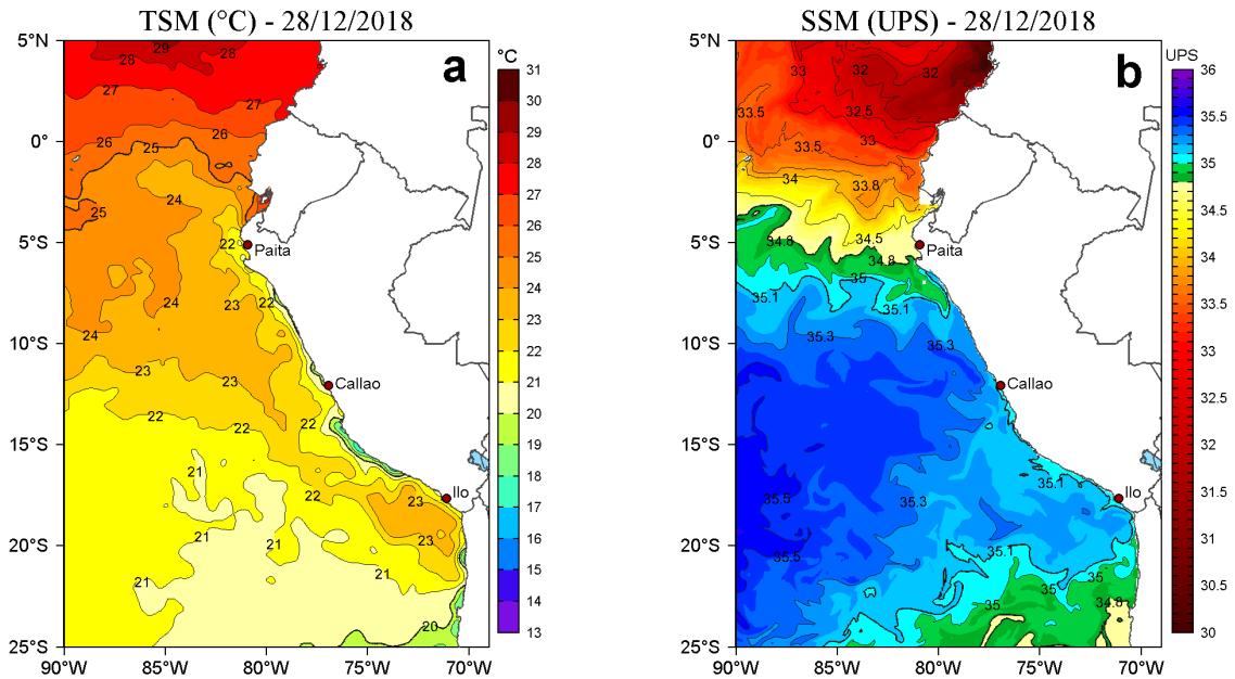
Figura 2. a) Temperatura superficial del mar (TSM, °C) y b) Salinidad superficial del mar (SSM, UPS) para el 28 de diciembre de 2018. Datos: OSTIA-UKMO-L4-GLOB-v2.0 (UK Met Office, 2012; Donlon et al, 2012) disponible en https://podaac.jpl.nasa.gov/dataset/OSTIA-UKMO-L4-GLOB-v2.0 para (a) y Hybrid Coordinate Ocean Model v. GOFS 3.1 (HYCOM; Halliwell et al., 1998; 2000; Bleck, 2001) para (b). Procesamiento: LHF/AFIOF/DGIOCC/IMARPE.
