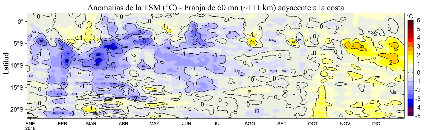
Figura 4. Variación promedio de las anomalías de la temperatura superficial del mar (TSM, °C) para una franja de 60 mn (~111 km) adyacente al litoral peruano para los últimos doce meses al 28 de diciembre de 2018. Datos: OSTIA-UKMO-L4-GLOB-v2.0 (UK Met. Office, 2012; Donlon et al, 2012) disponible en https://podaac.jpl.nasa.gov/dataset/OSTIA-UKMO-L4-GLOB-v2.0 ). Las anomalías se calcularon con respecto al periodo 2007-2016. Procesamiento: LHF/AFIOF/DGIOCC/IMARPE.
