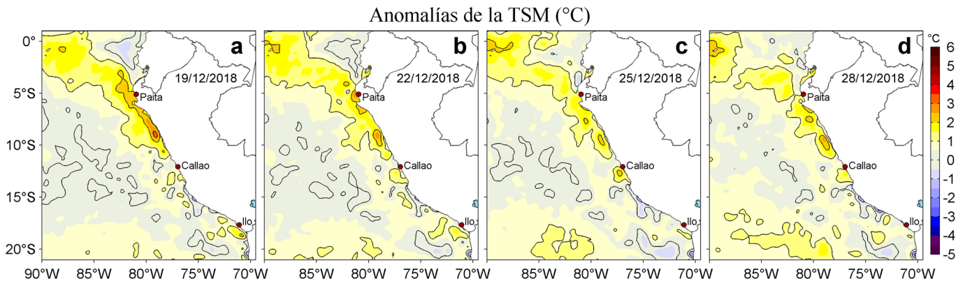
Figura 3. Anomalías de la temperatura superficial del mar (TSM, °C) para los días: a) 19, b) 22, c) 25 y d) 28 de diciembre de 2018. Las anomalías se calcularon respecto de la climatología para el periodo 2007-2016. Datos: OSTIA-UKMO-L4-GLOB-v2.0 (UK Met Office, 2012; Donlon et al, 2012). Procesamiento: LHF/AFIOF/DGIOCC/IMARPE.
