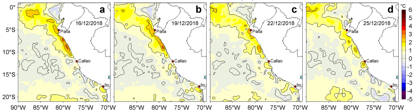
Figura 3. Anomalías de la temperatura superficial del mar (TSM, °C) para los días: a) 16, b) 19, c) 22 y d) 25 de diciembre de 2018. Las anomalías se calcularon respecto de la climatología para el periodo 2007-2016. Datos: OSTIA-UKMO-L4-GLOB-v2.0 (UK Met Office, 2012; Donlon et al, 2012). Procesamiento: LHF/AFIOF/DGIOCC/IMARPE.
