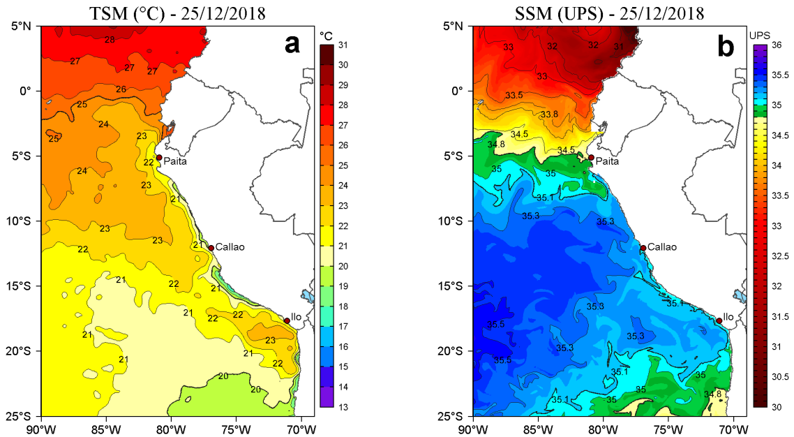
Figura 2. a) Temperatura superficial del mar (TSM, °C) y b) Salinidad superficial del mar (SSM, UPS) para el 25 de diciembre de 2018. Datos: OSTIA-UKMO-L4-GLOB-v2.0 (UK Met Office, 2012; Donlon et al, 2012) disponible en https://podaac.jpl.nasa.gov/dataset/OSTIA-UKMO-L4-GLOB-v2.0 para (a) y Hybrid Coordinate Ocean Model v. GOFS 3.1 (HYCOM; Halliwell et al., 1998; 2000; Bleck, 2001) para (b). Procesamiento: LHF/AFIOF/DGIOCC/IMARPE.
