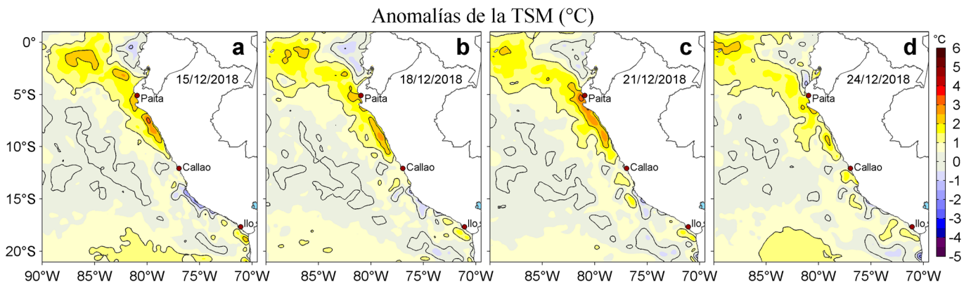
Figura 3. Anomalías de la temperatura superficial del mar (TSM, °C) para los días: a) 15, b) 18, c) 21 y d) 24 de diciembre de 2018. Las anomalías se calcularon respecto de la climatología para el periodo 2007-2016. Datos: OSTIA-UKMO-L4-GLOB-v2.0 (UK Met Office, 2012; Donlon et al, 2012). Procesamiento: LHF/AFIOF/DGIOCC/IMARPE.
