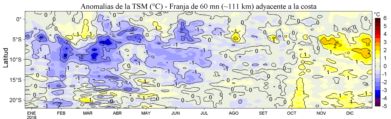
Figura 4. Variación promedio de las anomalías de la temperatura superficial del mar (TSM, °C) para una franja de 60 mn (~111 km) adyacente al litoral peruano para los últimos doce meses al 24 de diciembre de 2018. Datos: OSTIA-UKMO-L4-GLOB-v2.0 (UK Met. Office, 2012; Donlon et al, 2012) disponible en https://podaac.jpl.nasa.gov/dataset/OSTIA-UKMO-L4-GLOB-v2.0 ). Las anomalías se calcularon con respecto al periodo 2007-2016. Procesamiento: LHF/AFIOF/DGIOCC/IMARPE.
