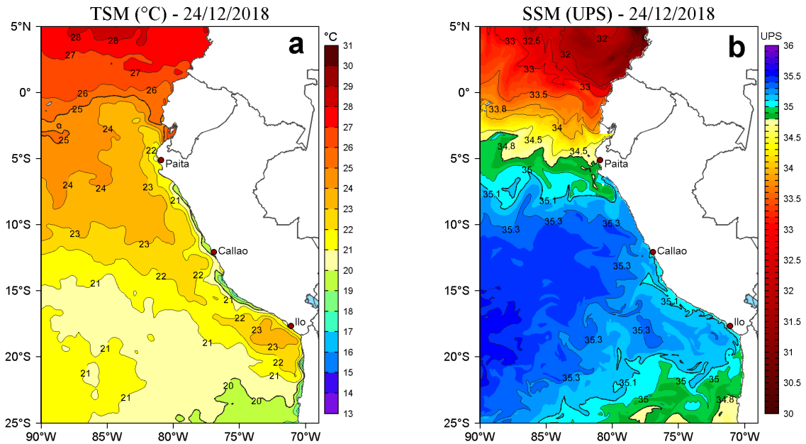
Figura 2. a) Temperatura superficial del mar (TSM, °C) y b) Salinidad superficial del mar (SSM, UPS) para el 24 de diciembre de 2018. Datos: OSTIA-UKMO-L4-GLOB-v2.0 (UK Met Office, 2012; Donlon et al, 2012) disponible en https://podaac.jpl.nasa.gov/dataset/OSTIA-UKMO-L4-GLOB-v2.0 para (a) y Hybrid Coordinate Ocean Model v. GOFS 3.1 (HYCOM; Halliwell et al., 1998; 2000; Bleck, 2001) para (b). Procesamiento: LHF/AFIOF/DGIOCC/IMARPE.
