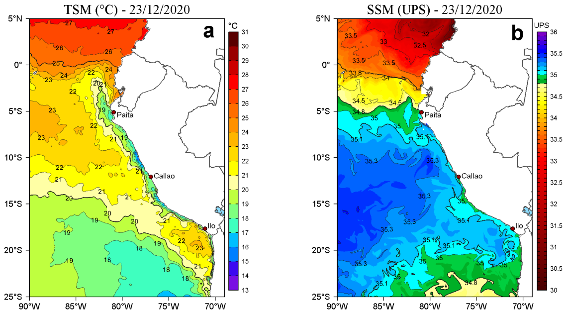
Figura 2. a) Temperatura superficial del mar (TSM, °C) y b) Salinidad superficial del mar (SSM, UPS), para el 23 de diciembre de 2020. Datos: OSTIA-UKMO-L4-GLOB-v2.0 (UK Met Office, 2012; Donlon et al, 2012) disponible en https://podaac.jpl.nasa.gov/dataset/OSTIA-UKMO-L4-GLOB-v2.0 para (a) y Hybrid Coordinate Ocean Model v. GOFS 3.1 (HYCOM; Halliwell et al., 1998; 2000; Bleck, 2001) para (b). Procesamiento: LHF/AFIOF/DGIOCC.
