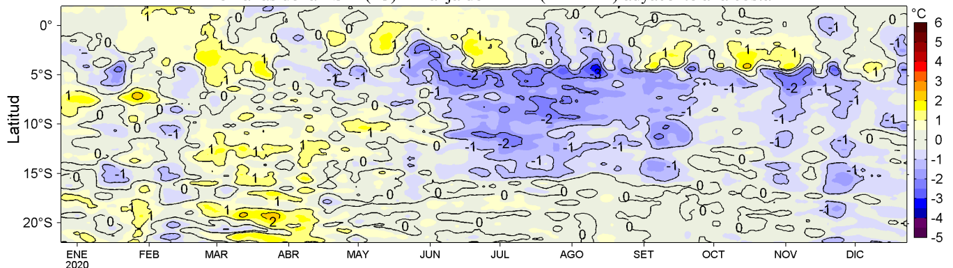
Figura 4. Variación promedio de las anomalías de la temperatura superficial del mar (TSM, °C) para una franja de 60 mn (~111 km) adyacente al litoral peruano para los últimos doce meses al 23 de diciembre de 2020. Datos: OSTIA-UKMO-L4-GLOB-v2.0 (UK Met. Office, 2012; Donlon et al, 2012) disponible en https://podaac.jpl.nasa.gov/dataset/OSTIA-UKMO-L4-GLOB-v2.0 . Las anomalías se calcularon con respecto al periodo 2007-2016. Procesamiento: LHF/AFIOF/DGIOCC.
