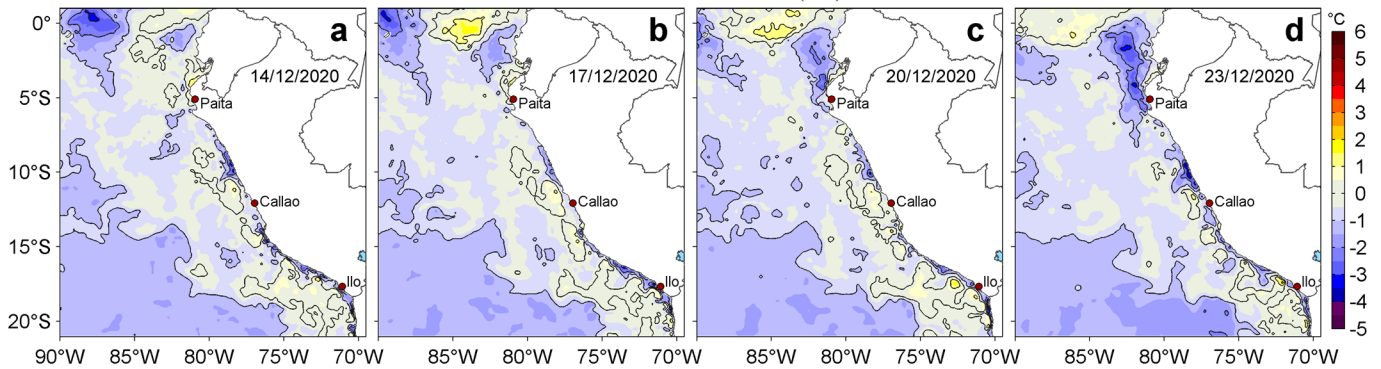
Figura 3. Anomalías de la temperatura superficial del mar (TSM, °C) para los días: a) 14, b) 17, c) 20 y d) 23 de diciembre de 2020. Las anomalías se calcularon respecto de la climatología para el periodo 2007-2016. Datos: OSTIA-UKMO-L4-GLOB-v2.0 (UK Met Office, 2012; Donlon et al, 2012). Procesamiento: LHF/AFIOF/DGIOCC.
