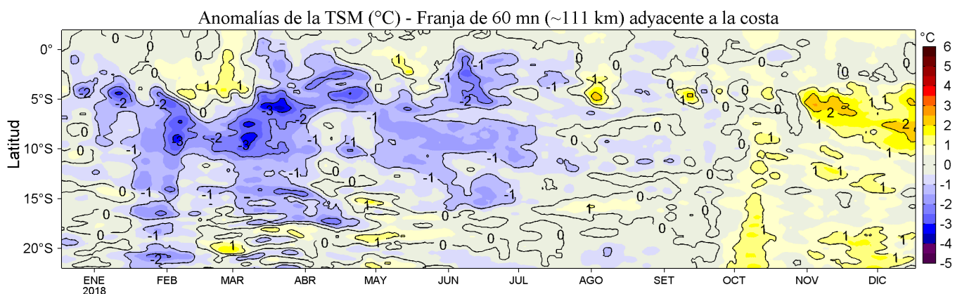
Figura 4. Variación promedio de las anomalías de la temperatura superficial del mar (°C) para una franja de 60 mn (~111 km) adyacente al litoral peruano para los últimos doce meses al 17 de diciembre de 2018. Datos: OSTIA-UKMO-L4-GLOB-v2.0 (UK Met. Office, 2012; Donlon et al, 2012) disponible en https://podaac.jpl.nasa.gov/dataset/OSTIA-UKMO-L4-GLOB-v2.0 . Las anomalías se calcularon con respecto al periodo 2007-2016. Procesamiento: LHF/AFIOF/DGIOCC/IMARPE.
