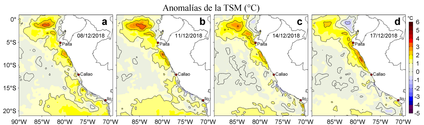
Figura 3. Anomalías de la temperatura superficial del mar (°C) para los días: a) 08, b) 11, c) 14 y d) 17 de diciembre de 2018. Las anomalías se calcularon respecto de la climatología para el periodo 2007-2016. Datos: OSTIA-UKMO-L4-GLOB-v2.0 (UK Met Office, 2012; Donlon et al, 2012). Procesamiento: LHF/AFIOF/DGIOCC/IMARPE.
