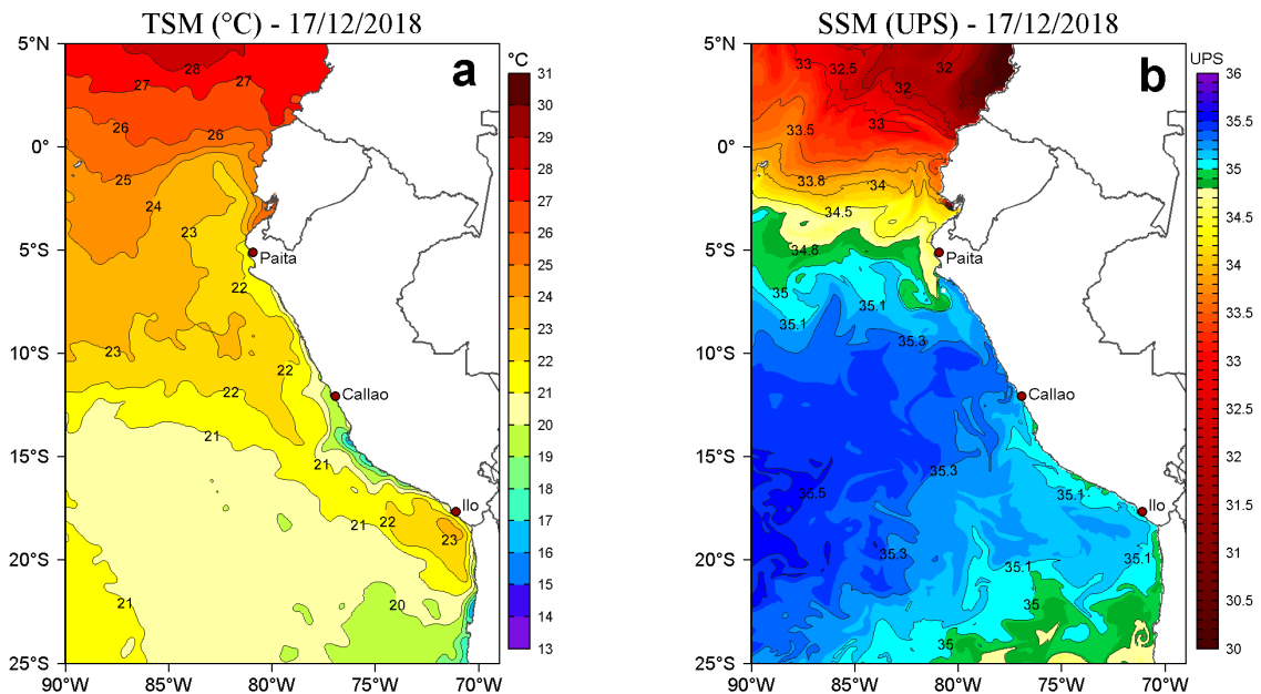
Figura 2. a) Temperatura superficial del mar (TSM, °C) y b) Salinidad superficial del mar (SSM, UPS) para el 17 de diciembre de 2018. Datos: OSTIA-UKMO-L4-GLOB-v2.0 (UK Met Office, 2012; Donlon et al, 2012) disponible en https://podaac.jpl.nasa.gov/dataset/OSTIA-UKMO-L4-GLOB-v2.0 para (a) y Hybrid Coordinate Ocean Model v. GOFS 3.1 (HYCOM; Halliwell et al., 1998; 2000; Bleck, 2001) para (b). Procesamiento: LHF/AFIOF/DGIOCC/IMARPE.
