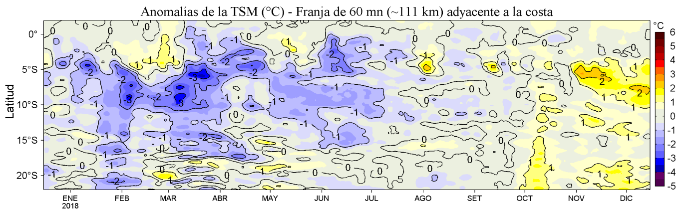
Figura 4. Variación promedio de las anomalías de la temperatura superficial del mar (TSM, °C) para una franja de 60 mn (~111 km) adyacente al litoral peruano para los últimos doce meses al 15 de diciembre de 2018. Datos: OSTIA-UKMO-L4-GLOB-v2.0 (UK Met. Office, 2012; Donlon et al, 2012) disponible en https://podaac.jpl.nasa.gov/dataset/OSTIA-UKMO-L4-GLOB-v2.0 ). Las anomalías se calcularon con respecto al periodo 2007-2016. Procesamiento: LHF/AFIOF/DGIOCC/IMARPE.
