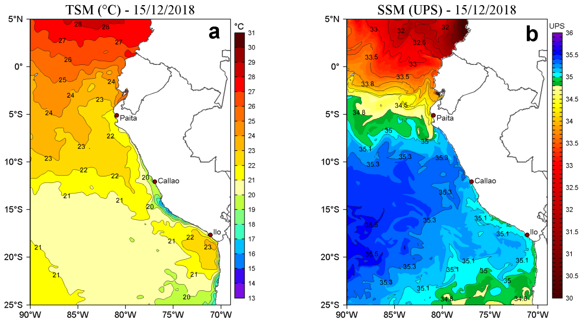
Figura 2. a) Temperatura superficial del mar (TSM, °C) y b) Salinidad superficial del mar (SSM, UPS) para el 15 de diciembre de 2018. Datos: OSTIA-UKMO-L4-GLOB-v2.0 (UK Met Office, 2012; Donlon et al, 2012) disponible en https://podaac.jpl.nasa.gov/dataset/OSTIA-UKMO-L4-GLOB-v2.0 para (a) y Hybrid Coordinate Ocean Model v. GOFS 3.1 (HYCOM; Halliwell et al., 1998; 2000; Bleck, 2001) para (b). Procesamiento: LHF/AFIOF/DGIOCC/IMARPE.
