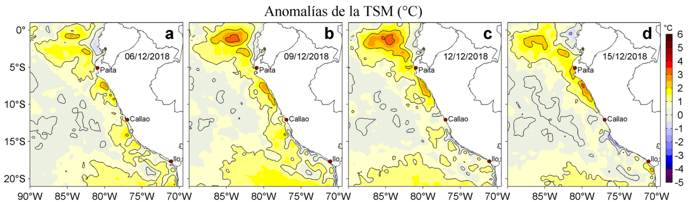
Figura 3. Anomalías de la temperatura superficial del mar (TSM, °C) para los días: a) 06, b) 09, c) 12 y d) 15 de diciembre de 2018. Las anomalías se calcularon respecto de la climatología para el periodo 2007-2016. Datos: OSTIA-UKMO-L4-GLOB-v2.0 (UK Met Office, 2012; Donlon et al, 2012). Procesamiento: LHF/AFIOF/DGIOCC/IMARPE.
