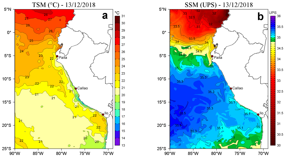
Figura 2. a) Temperatura superficial del mar (TSM, °C) y b) Salinidad superficial del mar (SSM, UPS) para el 13 de diciembre de 2018. Datos: OSTIA-UKMO-L4-GLOB-v2.0 (UK Met Office, 2012; Donlon et al, 2012) disponible en https://podaac.jpl.nasa.gov/dataset/OSTIA-UKMO-L4-GLOB-v2.0 para (a) y Hybrid Coordinate Ocean Model v. GOFS 3.1 (HYCOM; Halliwell et al., 1998; 2000; Bleck, 2001) para (b). Procesamiento: LHF/AFIOF/DGIOCC/IMARPE.
