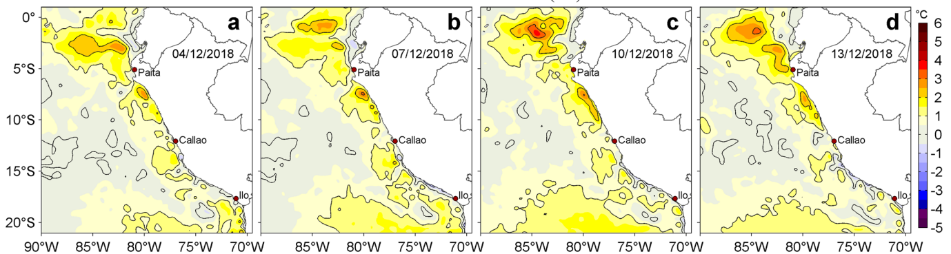
Figura 3. Anomalías de la temperatura superficial del mar (TSM, °C) para los días: a) 04, b) 07, c) 10 y d) 13 de diciembre de 2018. Las anomalías se calcularon respecto de la climatología para el periodo 2007-2016. Datos: OSTIA-UKMO-L4-GLOB-v2.0 (UK Met Office, 2012; Donlon et al, 2012). Procesamiento: LHF/AFIOF/DGIOCC/IMARPE.
