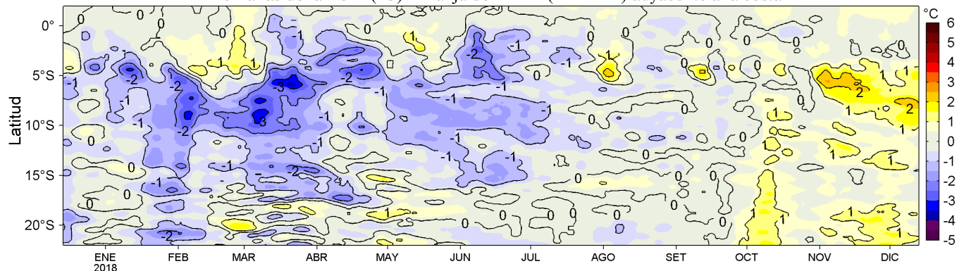
Figura 4. Variación promedio de las anomalías de la temperatura superficial del mar (TSM, °C) para una franja de 60 mn (~111 km) adyacente al litoral peruano para los últimos doce meses al 13 de diciembre de 2018. Datos: OSTIA-UKMO-L4-GLOB-v2.0 (UK Met. Office, 2012; Donlon et al, 2012) disponible en https://podaac.jpl.nasa.gov/dataset/OSTIA-UKMO-L4-GLOB-v2.0 ). Las anomalías se calcularon con respecto al periodo 2007-2016. Procesamiento: LHF/AFIOF/DGIOCC/IMARPE.
