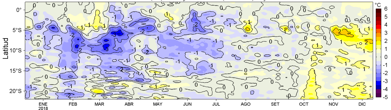
Figura 4. Variación promedio de las anomalías de la temperatura superficial del mar TSM (°C) para una franja de 60 mn (~111 km) adyacente al litoral peruano para los últimos doce meses al 12 de diciembre de 2018. Datos: OSTIA-UKMO-L4-GLOB-v2.0 (UK Met. Office, 2012; Donlon et al, 2012) disponible en https://podaac.jpl.nasa.gov/dataset/OSTIA-UKMO-L4-GLOB-v2.0 . Las anomalías se calcularon con respecto al periodo 2007-2016. Procesamiento: LHF/AFIOF/DGIOCC/IMARPE.
