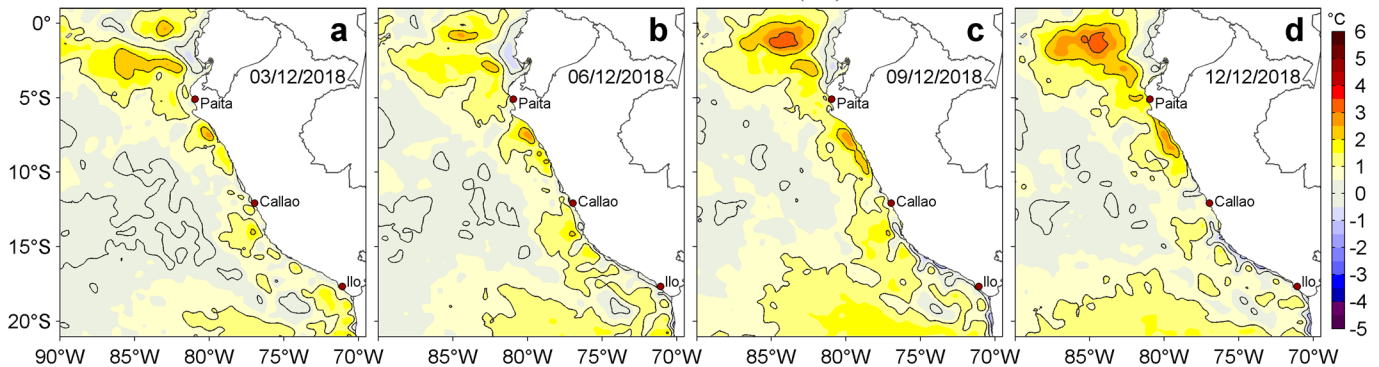
Figura 3. Anomalías de la temperatura superficial del mar (TSM, °C) para los días: a) 03, b) 06, c) 09 y d) 12 de diciembre de 2018. Las anomalías se calcularon respecto de la climatología para el periodo 2007-2016. Datos: OSTIA-UKMO-L4-GLOB-v2.0 (UK Met Office, 2012; Donlon et al, 2012). Procesamiento: LHF/AFIOF/DGIOCC/IMARPE.
