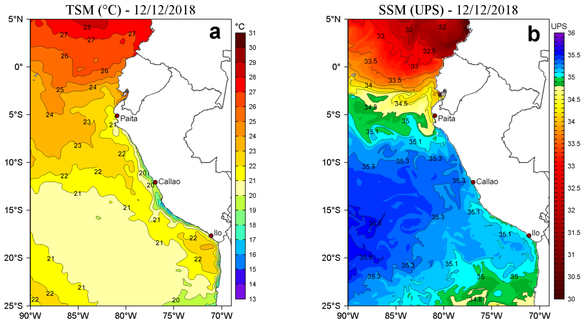
Figura 2. a) Temperatura superficial del mar (TSM, °C) y b) Salinidad superficial del mar (SSM, UPS) para el 12 de diciembre de 2018. Datos: OSTIA-UKMO-L4-GLOB-v2.0 (UK Met Office, 2012; Donlon et al, 2012) disponible en https://podaac.jpl.nasa.gov/dataset/OSTIA-UKMO-L4-GLOB-v2.0 para (a) y Hybrid Coordinate Ocean Model v. GOFS 3.1 (HYCOM; Halliwell et al., 1998; 2000; Bleck, 2001) para (b). Procesamiento: LHF/AFIOF/DGIOCC/IMARPE.
