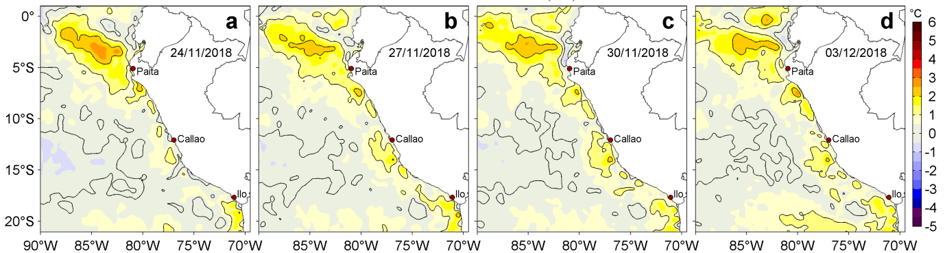
Figura 3. Anomalías de la temperatura superficial del mar TSM ( ^{\circ}\text{C} ) para los días: a) 24, b) 27 y c) 30 de noviembre y d) 03 de diciembre de 2018. Las anomalías se calcularon respecto de la climatología para el periodo 2007-2016. Datos: OSTIA-UKMO-L4-GLOB-v2.0 (UK Met Office, 2012; Donlon et al, 2012). Procesamiento: LHF/AFIOF/DGIOCC/IMARPE.
