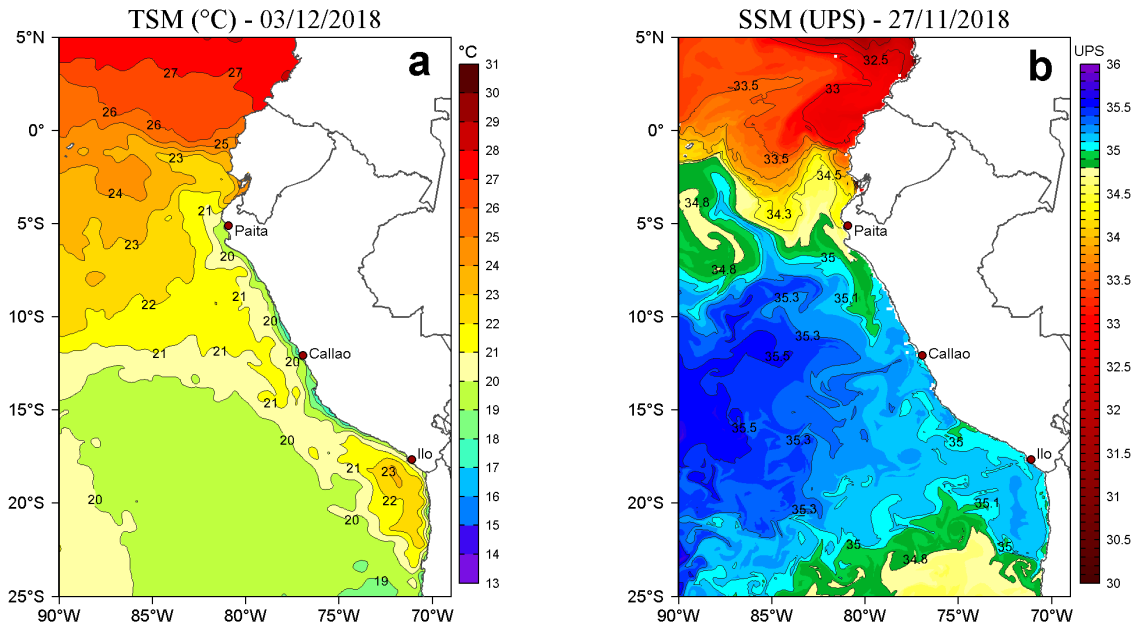
Figura 2. a) Temperatura superficial del mar TSM ( ^{\circ}\text{C} ) para el 03 de diciembre y b) Salinidad superficial del mar SSM (UPS) para el 27 de noviembre de 2018. Datos: OSTIA-UKMO-L4-GLOB-v2.0 (UK Met Office, 2012; Donlon et al, 2012) disponible en https://podaac.jpl.nasa.gov/dataset/OSTIA-UKMO-L4-GLOB-v2.0 para (a) y Hybrid Coordinate Ocean Model (HYCOM; Halliwell et al., 1998; 2000; Bleck, 2001) para (b). Procesamiento: LHF/AFIOF/DGIOCC/IMARPE.
