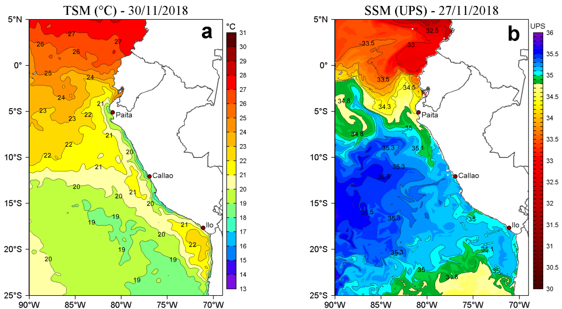
Figura 2. a) Temperatura superficial del mar (TSM, °C) para el 30 de noviembre y b) Salinidad superficial del mar (SSM, UPS) para el 27 de noviembre de 2018. Datos: OSTIA-UKMO-L4-GLOB-v2.0 (UK Met Office, 2012; Donlon et al, 2012) disponible en https://podaac.jpl.nasa.gov/dataset/OSTIA-UKMO-L4-GLOB-v2.0 ) para (a) y Hybrid Coordinate Ocean Model (HYCOM; Halliwell et al., 1998; 2000; Bleck, 2001) para (b). Procesamiento: LHF/AFIOF/DGIOCC/IMARPE.
