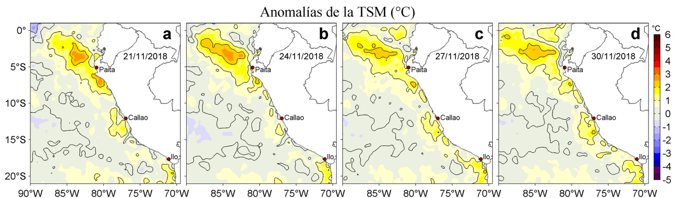
Figura 3. Anomalías de la temperatura superficial del mar (TSM, °C) para los días: a) 21, b) 24, c) 27 y d) 30 de noviembre de 2018. Las anomalías se calcularon respecto de la climatología para el periodo 2007-2016. Datos: OSTIA-UKMO-L4-GLOB-v2.0 (UK Met Office, 2012; Donlon et al, 2012). Procesamiento: LHF/AFIOF/DGIOCC/IMARPE.
