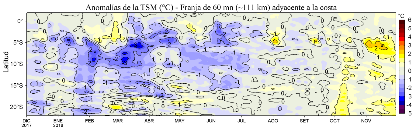
Figura 4. Variación promedio de las anomalías de la temperatura superficial del mar (TSM, °C) para una franja de 60 mn (~111 km) adyacente al litoral peruano para los últimos doce meses al 30 de noviembre de 2018. Datos: OSTIA-UKMO-L4-GLOB-v2.0 (UK Met. Office, 2012; Donlon et al, 2012) disponible en https://podaac.jpl.nasa.gov/dataset/OSTIA-UKMO-L4-GLOB-v2.0 ). Las anomalías se calcularon con respecto al periodo 2007-2016. Procesamiento: LHF/AFIOF/DGIOCC/IMARPE.
