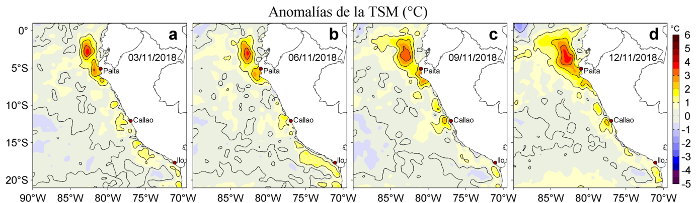
Figura 3. Anomalías de la temperatura superficial del mar (°C) para los días: a) 03, b) 06, c) 09 y d) 12 de noviembre de 2018. Las anomalías se calcularon respecto de la climatología para el periodo 2007-2016. Datos: OSTIA-UKMO-L4-GLOB-v2.0 (UK Met Office, 2012; Donlon et al, 2012). Procesamiento: LHF/AFIOF/DGIOCC/IMARPE.
