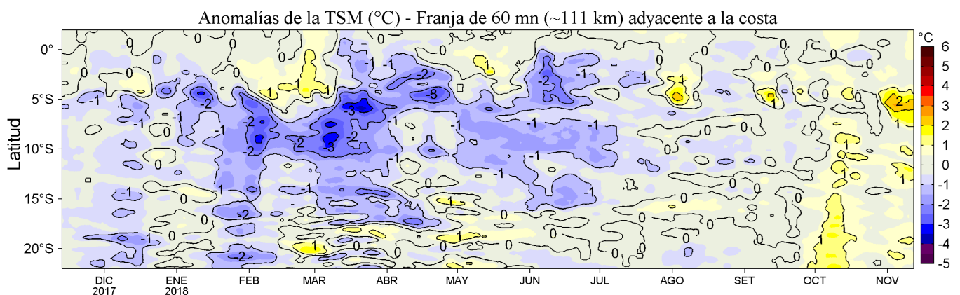
Figura 4. Variación promedio de las anomalías de la temperatura superficial del mar (°C) para una franja de 60 mn (~111 km) adyacente al litoral peruano para los últimos doce meses al 12 de noviembre de 2018. Datos: OSTIA-UKMO-L4-GLOB-v2.0 (UK Met. Office, 2012; Donlon et al, 2012) disponible en https://podaac.jpl.nasa.gov/dataset/OSTIA-UKMO-L4-GLOB-v2.0 ). Las anomalías se calcularon con respecto al periodo 2007-2016. Procesamiento: LHF/AFIOF/DGIOCC/IMARPE.
