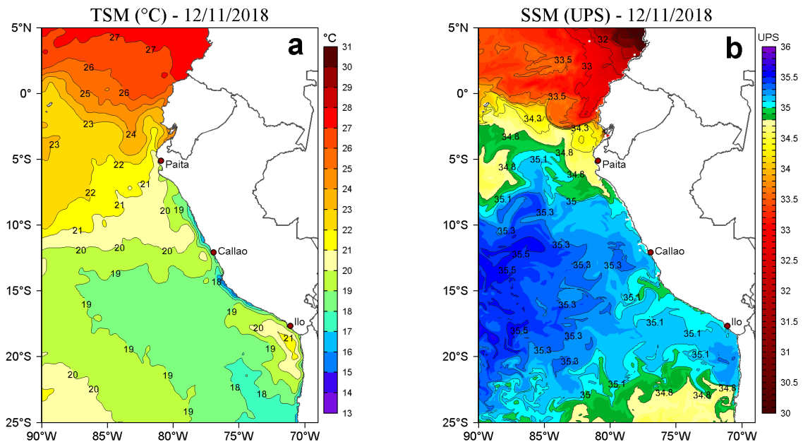
Figura 2. a) Temperatura superficial del mar (°C) y b) Salinidad superficial del mar (SSM, UPS) para el 12 de noviembre de 2018. Datos: OSTIA-UKMO-L4-GLOB-v2.0 (UK Met Office, 2012; Donlon et al, 2012) disponible en https://podaac.jpl.nasa.gov/dataset/OSTIA-UKMO-L4-GLOB-v2.0 ) para (a) y Hybrid Coordinate Ocean Model (HYCOM; Halliwell et al., 1998; 2000; Bleck, 2001) para (b). Procesamiento: LHF/AFIOF/DGIOCC/IMARPE.
