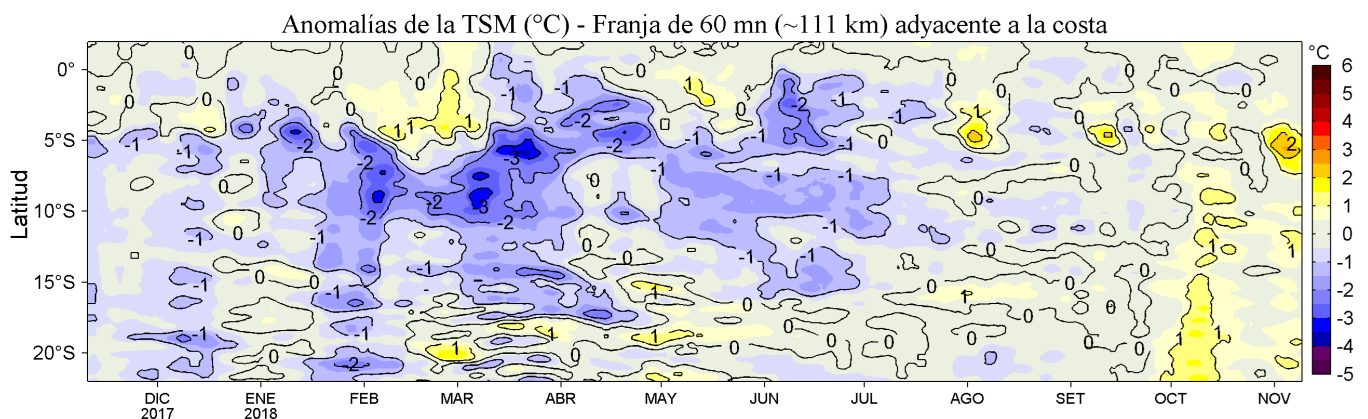
Figura 4. Variación promedio de las anomalías de la temperatura superficial del mar TSM (°C) para una franja de 60 mn (~111 km) adyacente al litoral peruano para los últimos doce meses al 09 de noviembre de 2018. Datos: OSTIA-UKMO-L4-GLOB-v2.0 (UK Met. Office, 2012; Donlon et al, 2012) disponible en https://podaac.jpl.nasa.gov/dataset/OSTIA-UKMO-L4-GLOB-v2.0 ). Las anomalías se calcularon con respecto al periodo 2007-2016. Procesamiento: LHFM/AFIOF/DGIOCC/IMARPE.
