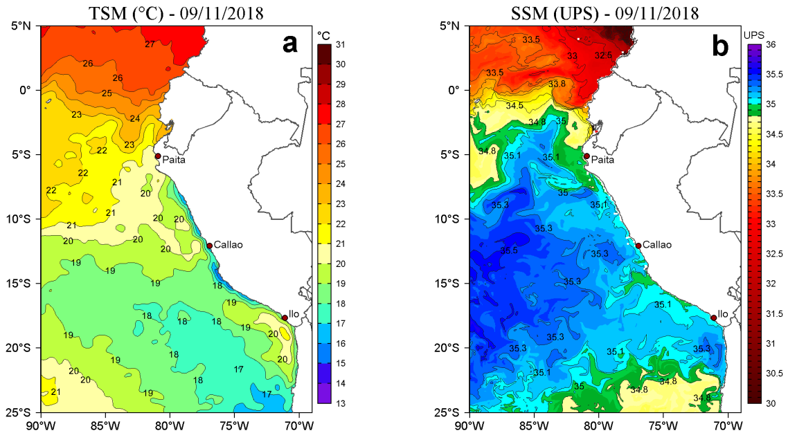
Figura 2. a) Temperatura superficial del mar (TSM, °C) y b) Salinidad superficial del mar (SSM, UPS) para el 09 de noviembre de 2018. Datos: OSTIA-UKMO-L4-GLOB-v2.0 (UK Met Office, 2012; Donlon et al, 2012) disponible en https://podaac.jpl.nasa.gov/dataset/OSTIA-UKMO-L4-GLOB-v2.0 para (a) y Hybrid Coordinate Ocean Model (HYCOM; Halliwell et al., 1998; 2000; Bleck, 2001) para (b). Procesamiento: LHFM/AFIOF/DGIOCC/IMARPE.
