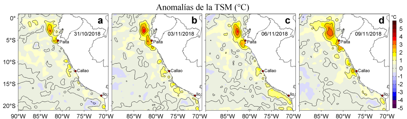
Figura 3. Anomalías de la temperatura superficial del mar (TSM, °C) para los días: a) 31 de octubre y b) 03, c) 06 y d) 09 de noviembre de 2018. Las anomalías se calcularon respecto de la climatología para el periodo 2007-2016. Datos: OSTIA-UKMO-L4-GLOB-v2.0 (UK Met Office, 2012; Donlon et al, 2012). Procesamiento: LHFM/AFIOF/DGIOCC/IMARPE.
