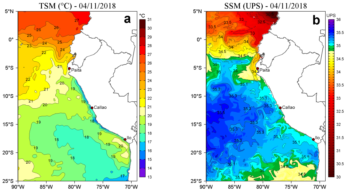
Figura 2. a) Temperatura superficial del mar TSM ( ^{\circ}\text{C} ) y b) Salinidad superficial del mar SSM (UPS) para el 04 de noviembre de 2018. Datos: OSTIA-UKMO-L4-GLOB-v2.0 (UK Met Office, 2012; Donlon et al, 2012) disponible en https://podaac.jpl.nasa.gov/dataset/OSTIA-UKMO-L4-GLOB-v2.0 ) para (a) y Hybrid Coordinate Ocean Model (HYCOM; Halliwell et al., 1998; 2000; Bleck, 2001) para (b). Procesamiento: LHFH/AFIOF/DGIOCC/IMARPE.
