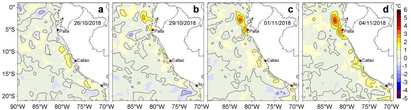
Figura 3. Anomalías de la temperatura superficial del mar TSM ( ^{\circ}\text{C} ) para los días: a) 26 y b) 29 de octubre, c) 01 y d) 04 de noviembre de 2018. Las anomalías se calcularon respecto de la climatología para el periodo 2007-2016. Datos: OSTIA-UKMO-L4-GLOB-v2.0 (UK Met Office, 2012; Donlon et al, 2012). Procesamiento: LHFH/AFIOF/DGIOCC/IMARPE.
