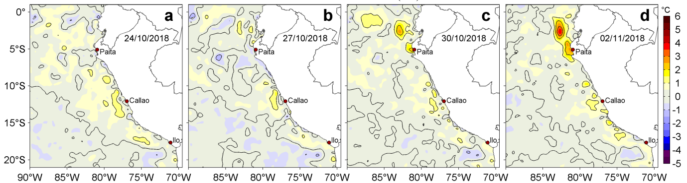
Figura 3. Anomalías de la temperatura superficial del mar TSM (°C) para los días: a) 24, b) 27 y c) 30 de octubre y d) 02 de noviembre de 2018. Las anomalías se calcularon respecto de la climatología para el periodo 2007-2016. Datos: OSTIA-UKMO-L4-GLOB-v2.0 (UK Met Office, 2012; Donlon et al, 2012). Procesamiento: LHFH/AFIOF/DGIOCC/IMARPE.
