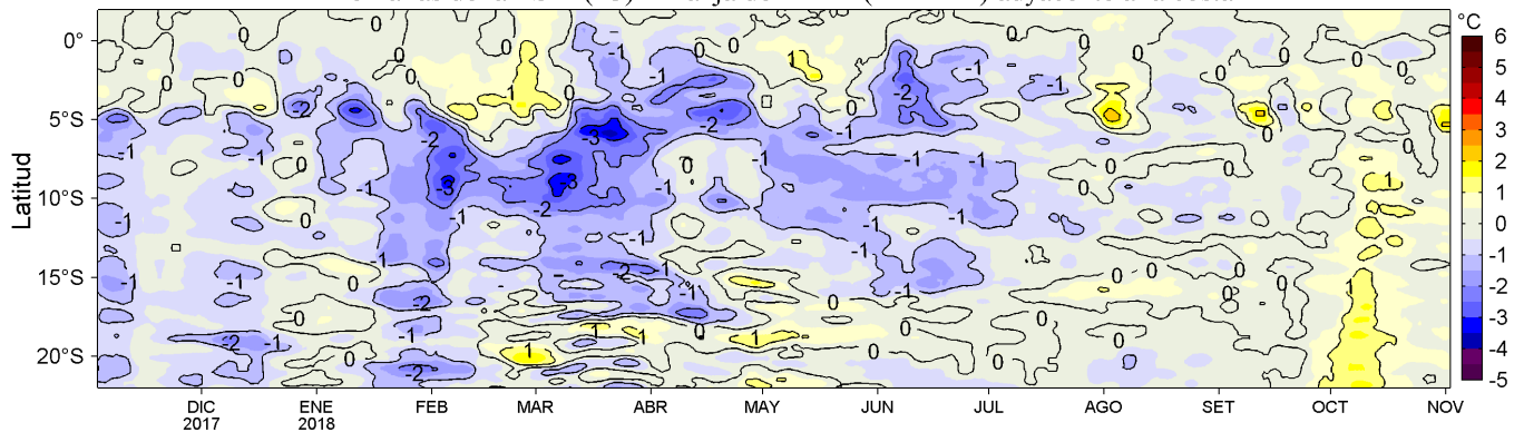
Figura 4. Variación promedio de las anomalías de la temperatura superficial del mar TSM (°C) para una franja de 60 mn (~111 km) adyacente al litoral peruano para los últimos doce meses al 02 de noviembre de 2018. Datos: OSTIA-UKMO-L4-GLOB-v2.0 (UK Met. Office, 2012; Donlon et al, 2012) disponible en https://podaac.jpl.nasa.gov/dataset/OSTIA-UKMO-L4-GLOB-v2.0 . Las anomalías se calcularon con respecto al periodo 2007-2016. Procesamiento: LHFH/AFIOF/DGIOCC/IMARPE.
