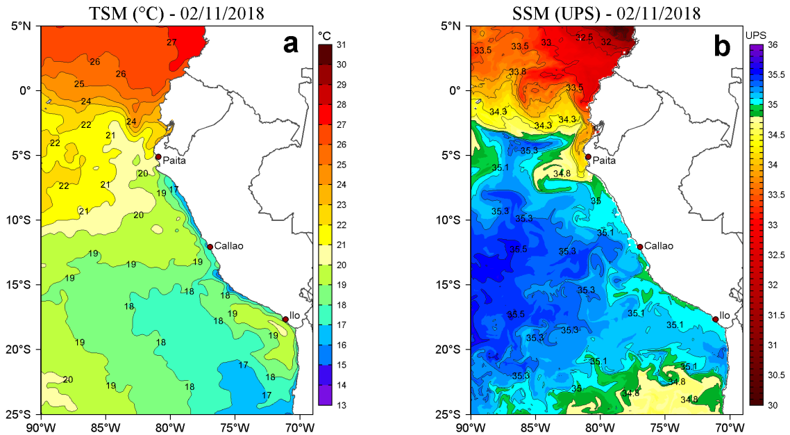
Figura 2. a) Temperatura superficial del mar TSM (°C) y b) Salinidad superficial del mar SSM (UPS) para el 02 de noviembre de 2018. Datos: OSTIA-UKMO-L4-GLOB-v2.0 (UK Met Office, 2012; Donlon et al, 2012) disponible en https://podaac.jpl.nasa.gov/dataset/OSTIA-UKMO-L4-GLOB-v2.0 para (a) y Hybrid Coordinate Ocean Model (HYCOM; Halliwell et al., 1998; 2000; Bleck, 2001) para (b). Procesamiento: LHFH/AFIOF/DGIOCC/IMARPE.
