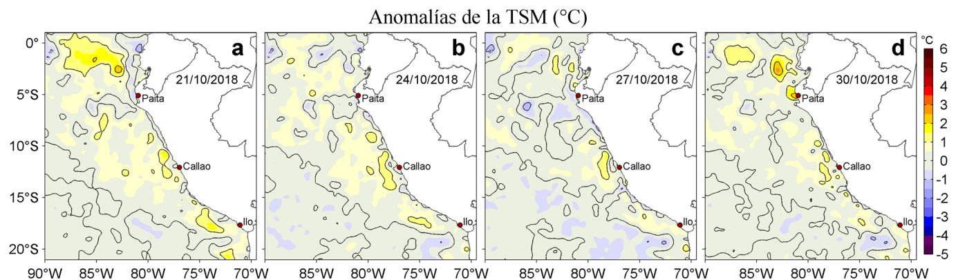
Figura 3. Anomalías de la temperatura superficial del mar (TSM, °C) para los días: a) 21, b) 24, c) 27 y d) 30 de octubre de 2018. Las anomalías se calcularon respecto de la climatología para el periodo 2007-2016. Datos: OSTIA-UKMO-L4-GLOB-v2.0 (UK Met Office, 2012; Donlon et al, 2012). Procesamiento: LHF/AFIOF/DGIOCC/IMARPE.
