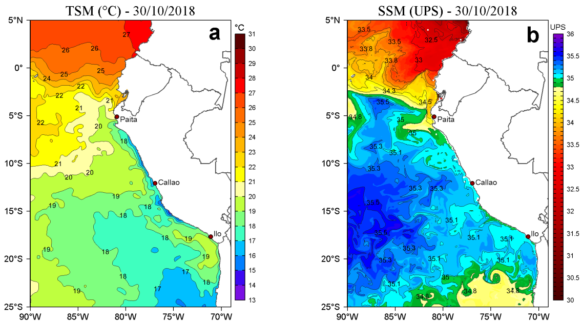
Figura 2. a) Temperatura superficial del mar (TSM, °C) y b) Salinidad superficial del mar (SSM, UPS) para el 30 de octubre de 2018. Datos: OSTIA-UKMO-L4-GLOB-v2.0 (UK Met Office, 2012; Donlon et al, 2012) disponible en https://podaac.jpl.nasa.gov/dataset/OSTIA-UKMO-L4-GLOB-v2.0 ) para (a) y Hybrid Coordinate Ocean Model (HYCOM; Halliwell et al., 1998; 2000; Bleck, 2001) para (b). Procesamiento: LHF/AFIOF/DGIOCC/IMARPE.
