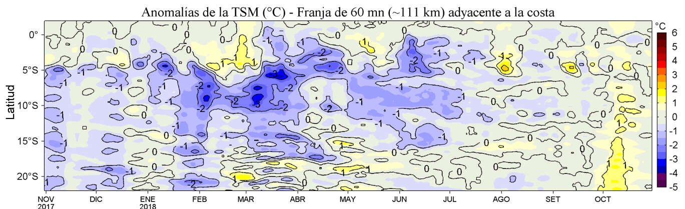
Figura 4. Variación promedio de las anomalías de la temperatura superficial del mar (TSM, °C) para una franja de 60 mn (~111 km) adyacente al litoral peruano para los últimos doce meses al 30 de octubre de 2018. Datos: OSTIA-UKMO-L4-GLOB-v2.0 (UK Met. Office, 2012; Donlon et al, 2012) disponible en https://podaac.jpl.nasa.gov/dataset/OSTIA-UKMO-L4-GLOB-v2.0 ). Las anomalías se calcularon con respecto al periodo 2007-2016. Procesamiento: LHF/AFIOF/DGIOCC/IMARPE.
