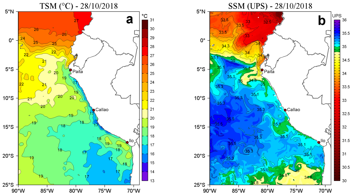
Figura 2. a) Temperatura superficial del mar (TSM, °C) y b) Salinidad superficial del mar (SSM, UPS) para el 28 de octubre de 2018. Datos: OSTIA-UKMO-L4-GLOB-v2.0 (UK Met Office, 2012; Donlon et al, 2012) disponible en https://podaac.jpl.nasa.gov/dataset/OSTIA-UKMO-L4-GLOB-v2.0 ) para (a) y Hybrid Coordinate Ocean Model (HYCOM; Halliwell et al., 1998; 2000; Bleck, 2001) para (b). Procesamiento: LHF/AFIOF/DGIOCC/IMARPE.
