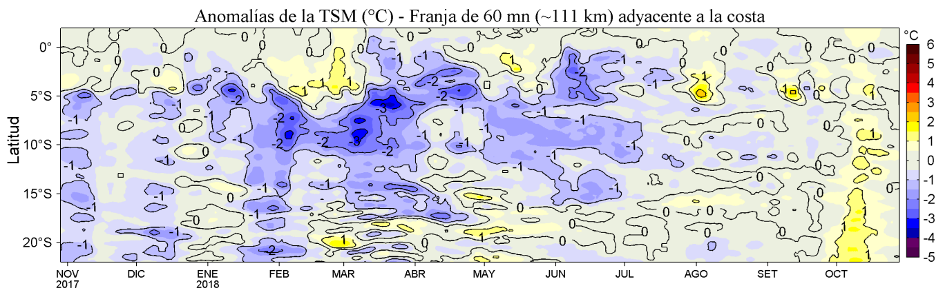
Figura 4. Variación promedio de las anomalías de la temperatura superficial del mar (TSM, °C) para una franja de 60 mn (~111 km) adyacente al litoral peruano para los últimos doce meses al 28 de octubre de 2018. Datos: OSTIA-UKMO-L4-GLOB-v2.0 (UK Met. Office, 2012; Donlon et al, 2012) disponible en https://podaac.jpl.nasa.gov/dataset/OSTIA-UKMO-L4-GLOB-v2.0 ). Las anomalías se calcularon con respecto al periodo 2007-2016. Procesamiento: LHF/AFIOF/DGIOCC/IMARPE.
