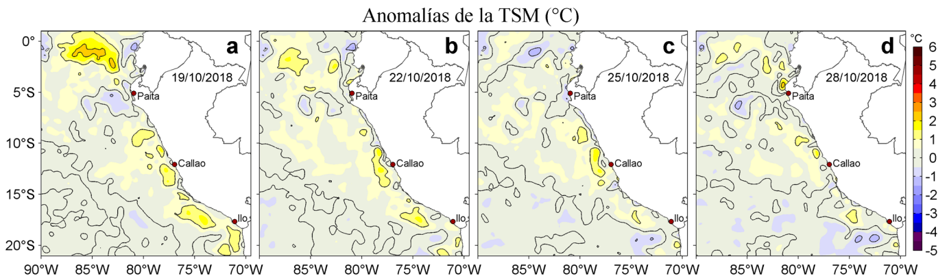
Figura 3. Anomalías de la temperatura superficial del mar (TSM, °C) para los días: a) 19, b) 22, c) 25 y d) 28 de octubre de 2018. Las anomalías se calcularon respecto de la climatología para el periodo 2007-2016. Datos: OSTIA-UKMO-L4-GLOB-v2.0 (UK Met Office, 2012; Donlon et al, 2012). Procesamiento: LHF/AFIOF/DGIOCC/IMARPE.
