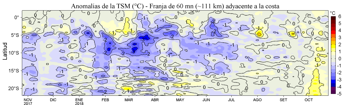
Figura 4. Variación promedio de las anomalías de la temperatura superficial del mar (TSM, °C) para una franja de 60 mn (~111 km) adyacente al litoral peruano para los últimos doce meses al 24 de octubre de 2018. Datos: OSTIA-UKMO-L4-GLOB-v2.0 (UK Met. Office, 2012; Donlon et al, 2012) disponible en https://podaac.jpl.nasa.gov/dataset/OSTIA-UKMO-L4-GLOB-v2.0 ). Las anomalías se calcularon con respecto al periodo 2007-2016. Procesamiento: LHF/AFIOF/DGIOCC/IMARPE.
