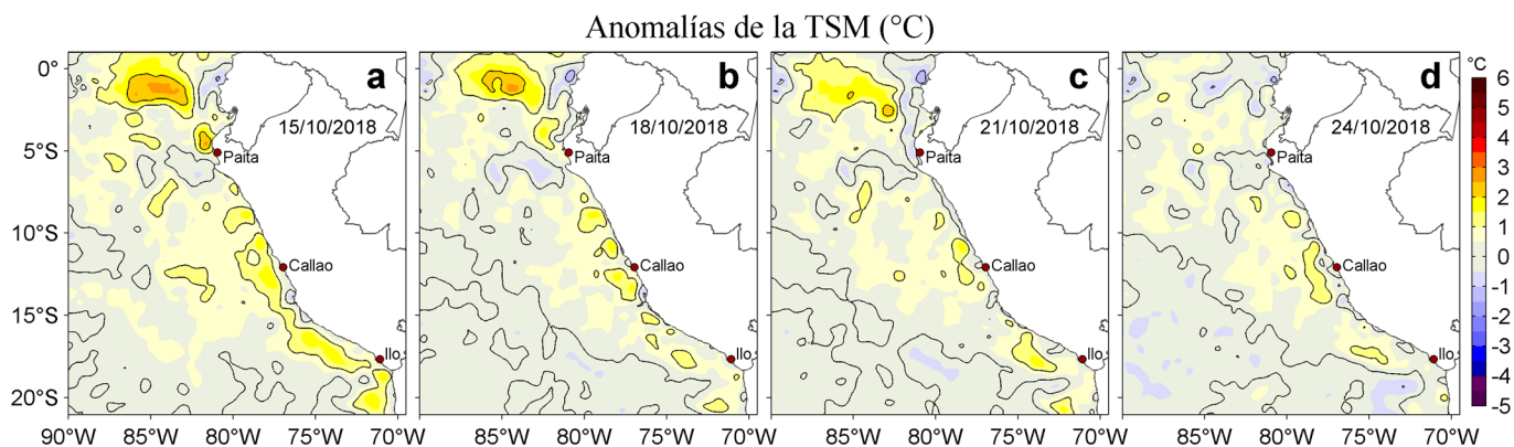
Figura 3. Anomalías de la temperatura superficial del mar (TSM, °C) para los días: a) 15, b) 18, c) 21 y d) 24 de octubre de 2018. Las anomalías se calcularon respecto de la climatología para el periodo 2007-2016. Datos: OSTIA-UKMO-L4-GLOB-v2.0 (UK Met Office, 2012; Donlon et al, 2012). Procesamiento: LHF/AFIOF/DGIOCC/IMARPE.
