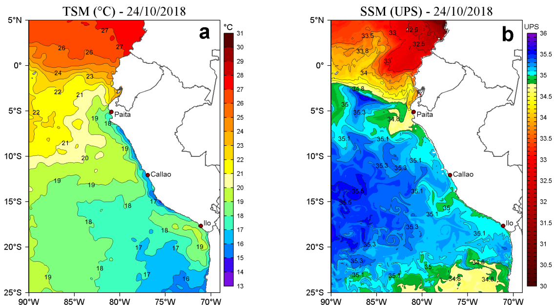
Figura 2. a) Temperatura superficial del mar (TSM, °C) y b) Salinidad superficial del mar (SSM, UPS) para el 24 de octubre de 2018. Datos: OSTIA-UKMO-L4-GLOB-v2.0 (UK Met Office, 2012; Donlon et al, 2012) disponible en https://podaac.jpl.nasa.gov/dataset/OSTIA-UKMO-L4-GLOB-v2.0 ) para (a) y Hybrid Coordinate Ocean Model (HYCOM; Halliwell et al., 1998; 2000; Bleck, 2001) para (b). Procesamiento: LHF/AFIOF/DGIOCC/IMARPE.
